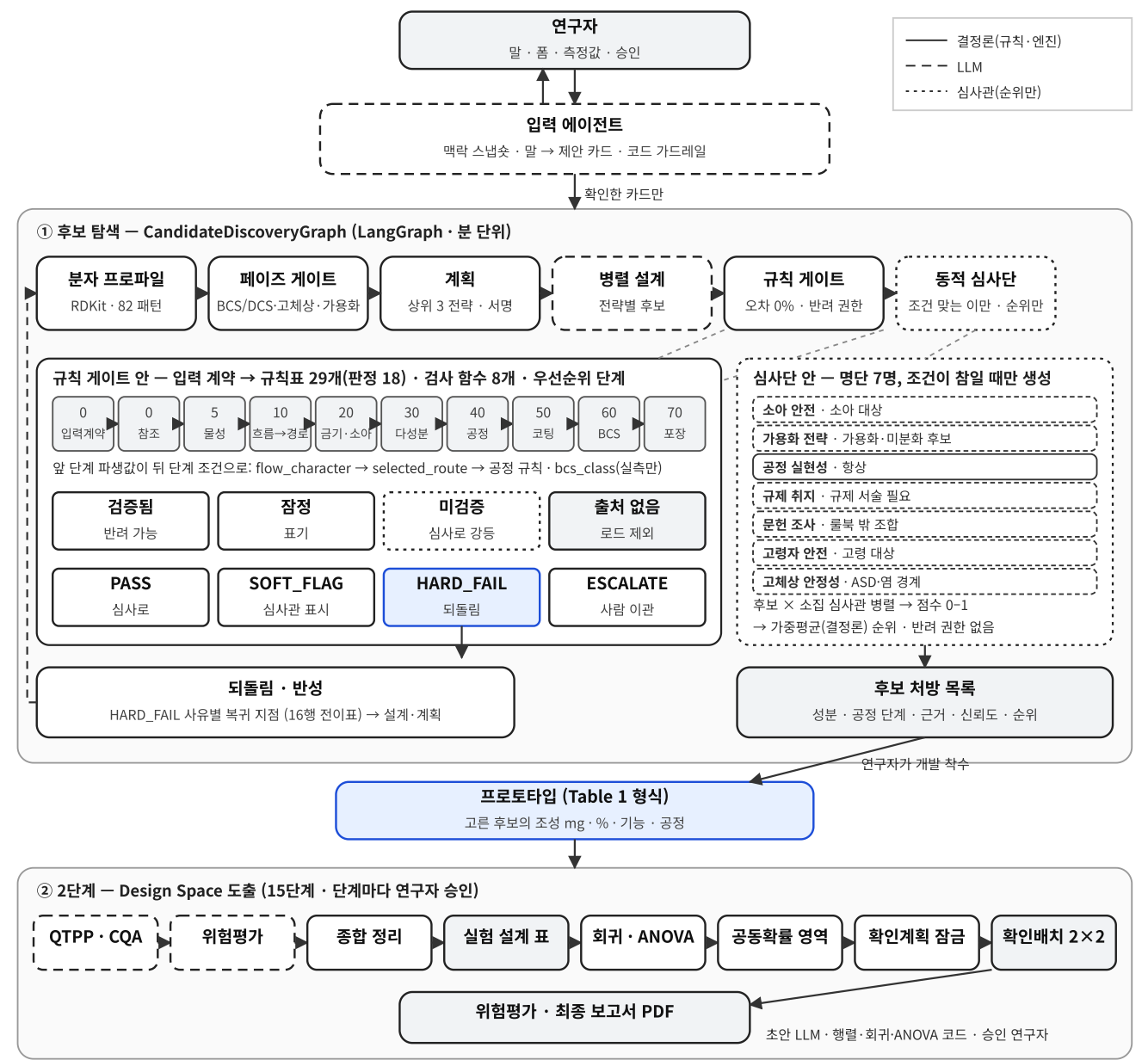
그림 1. 전체 구조. 연구자와 두 그래프 사이에 입력 에이전트가 있고, 두 단계는 내부 상태를 공유하지 않은 채 연구자가 고른 후보의 처방(프로토타입) 하나로만 연결된다. ① 안의 두 확대 상자는 규칙 게이트(우선순위 단계, 근거 상태별 권한, 판정별 경로 — 그림 4)와 동적 심사단(명단 7명과 소집 조건, 순위만 매기는 합의 — 그림 6)의 내부다. 선 모양은 담당 주체를 나타낸다(실선: 결정론 규칙·엔진, 파선: LLM, 점선: 순위만 매기는 심사관).
