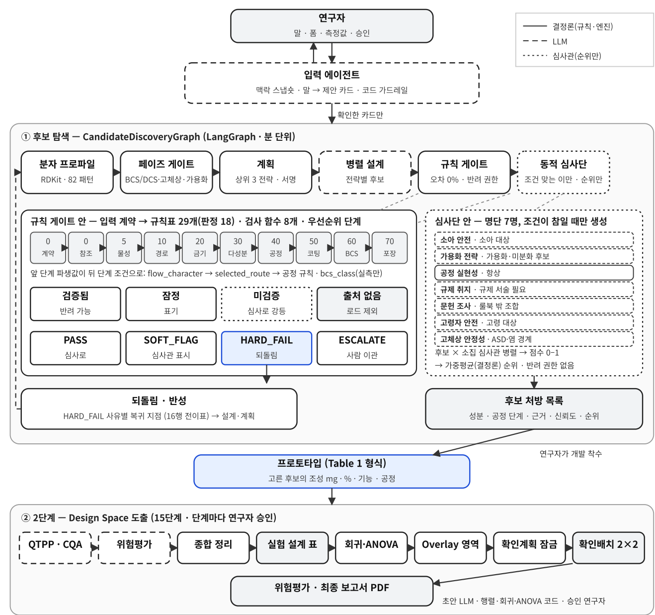
그림 2. 구성 요소 상세. 입력 에이전트가 연구자와 두 그래프 사이에 있고, 두 단계는 연구자가 선택한 후보의 처방(프로토타입) 하나로만 연결된다. ① 안의 두 확대 상자는 규칙 게이트(그림 5)와 동적 심사단(그림 7)의 내부 구조이다. 선 모양은 담당 주체를 나타낸다(실선: 결정론, 파선: LLM, 점선: 순위만 매기는 심사관).
