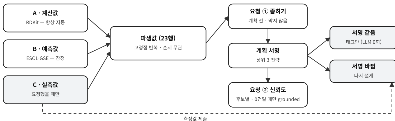
그림 4. 값의 세 계층과 비차단 실험 요청. 측정값이 들어오면 그래프를 다시 돌리지 않고 결정된 계층만 재계산하며, 계획 서명이 같으면 신뢰도 태그만 갱신한다.
