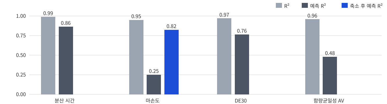
그림 8. 반응별 적합도. 마손도의 전체 이차모형은 R^2 0.95이나 예측 R^2 가 0.25로 과적합 flag(MV006)가 서고, 계층성을 지닌 선형 축소 후 예측 R^2 0.82로 회복했다. 함량균일성(예측 R^2 0.48)도 flag가 서며, 데모에서는 사유를 기록하고 수용했다. 잔차 자유도는 이차모형 5, 선형 11.
