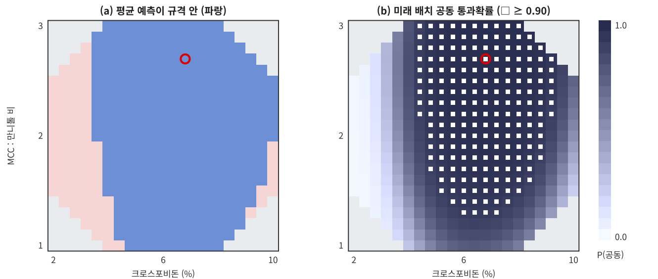
그림 9. 혼합 시간 12.5분 단면(설정점을 지나는 면, 엔진 계산 격자 21 \times 21 ). (a) 평균 예측만 보면 이 면의 지지 영역 중 79%가 규격 안이지만, (b) 미래 배치의 공동 통과확률 \geq 0.90 (흰 점)을 요구하면 50%만 남는다. 전체 격자에서 미달 점의 대부분은 DE30이 결정한다(표 4). 회색은 설계점 convex hull 밖(외삽), 빨간 원은 권장 설정점.
