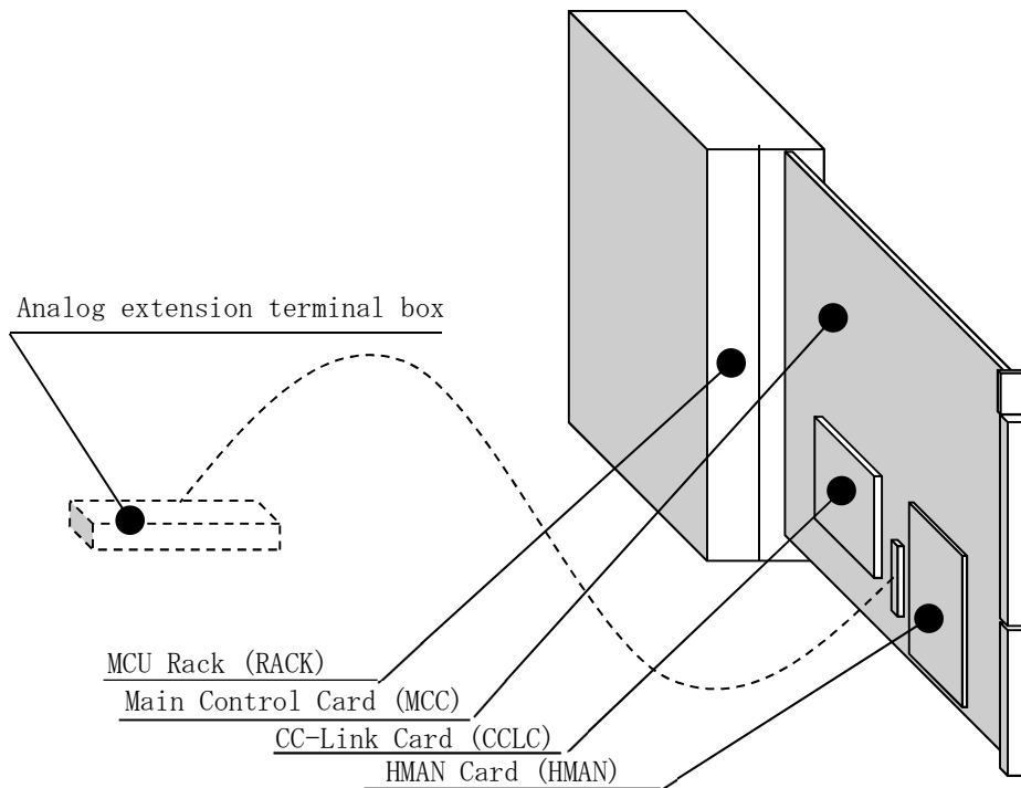
圖 3.2.2 MCU 硬體組成圖 (1)
