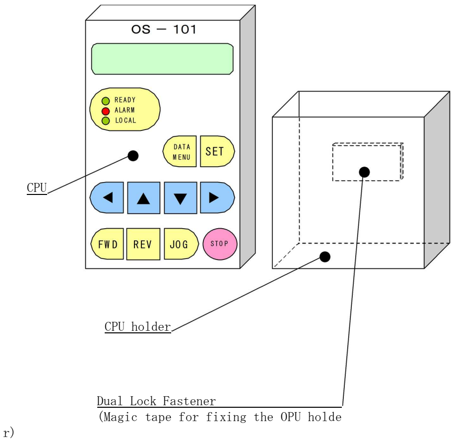
圖 3. 2. 6 OPU 硬體組成圖
