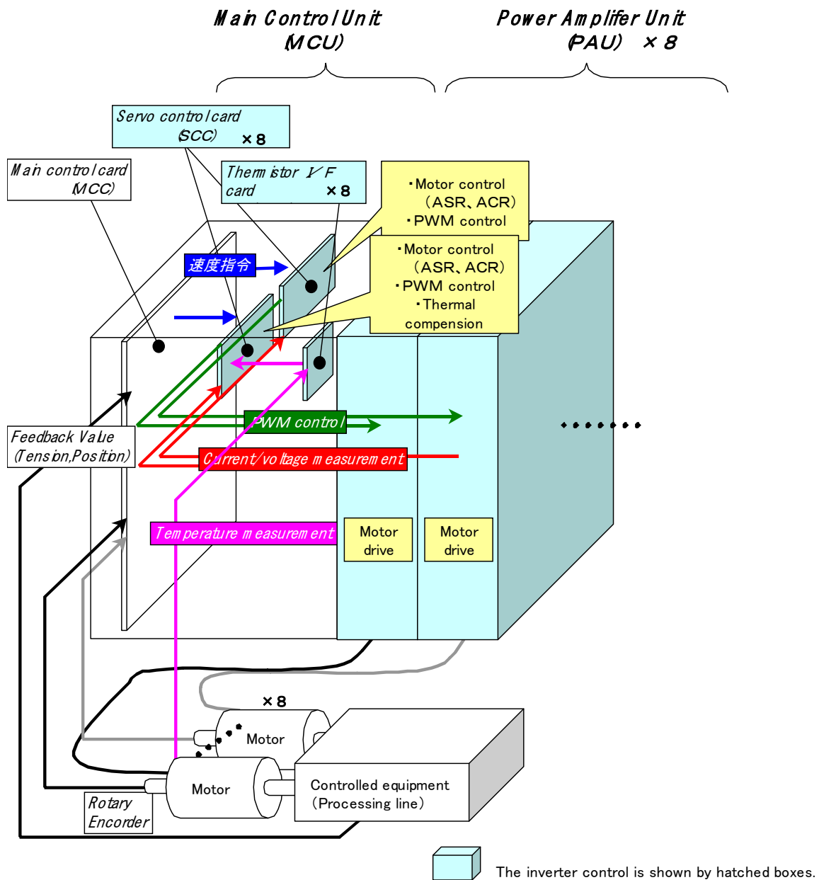
圖 3.1.1 逆變器控制原理圖
