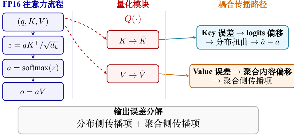
图 3-1 注意力误差的两条耦合传播路径及其精确代数分解。左侧为 FP16 attention flow，中部为量化扰动，右侧为由 Key 与 Value 误差分别触发的两条传播路径，底部标出输出误差对应的两类传播项。
