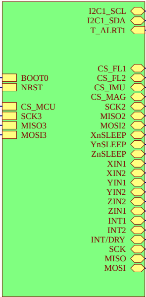
AOCS_MCU_446 MCU.SchDoc
