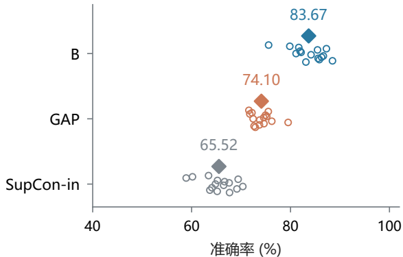
a Rank-1
