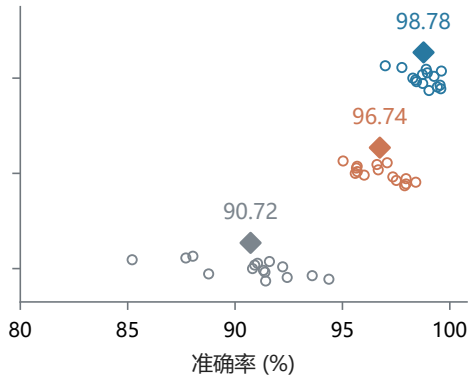
b Rank-5
