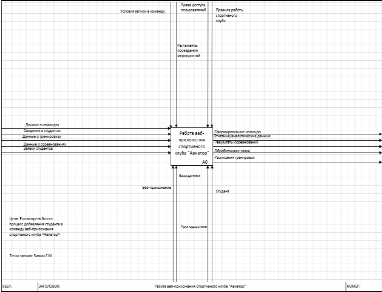
Контекстная диаграмма IDEF0
