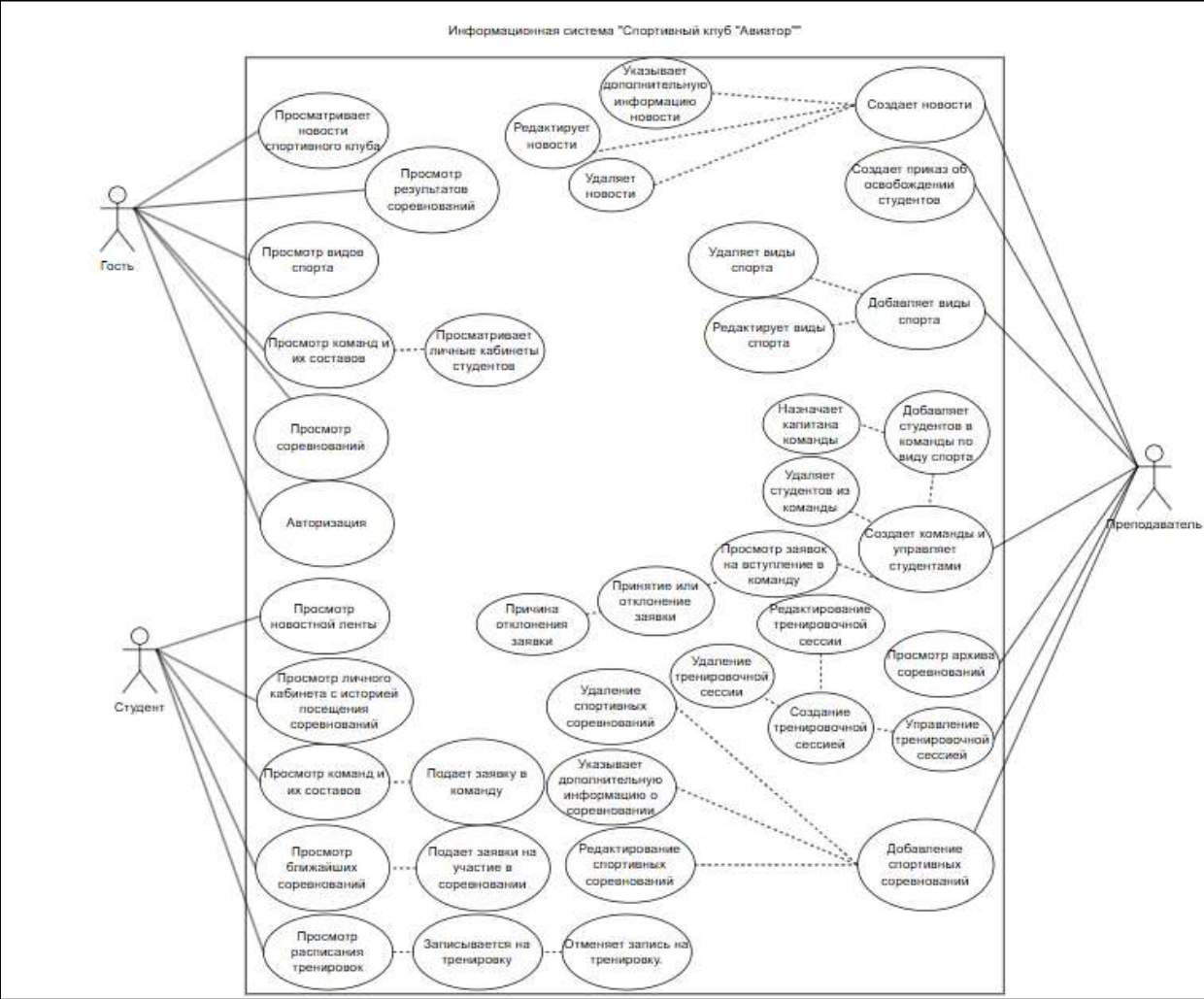
Диаграмма прецедентов
