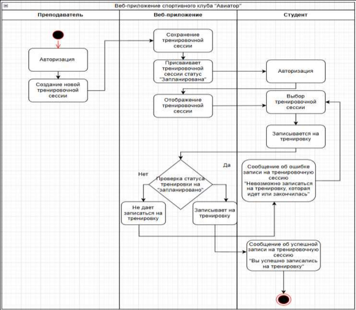
Диаграмма деятельности
