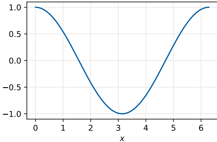
\cos(x)
