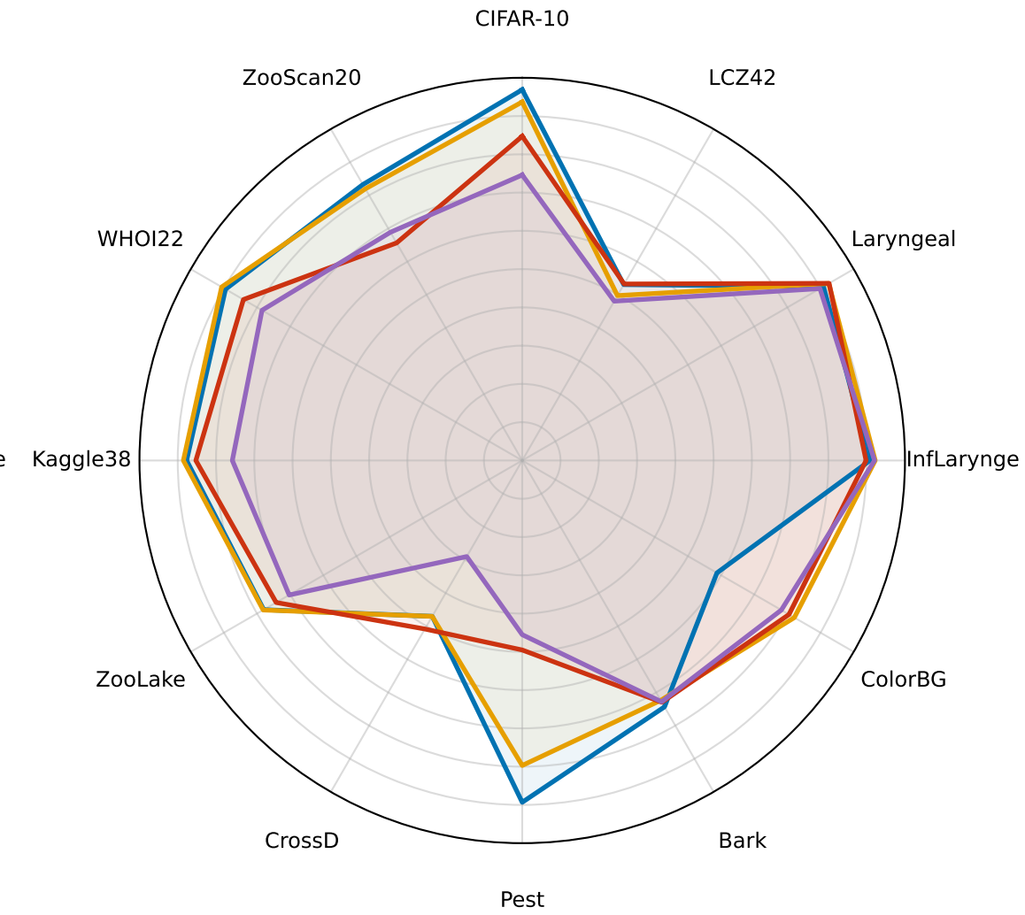
ViT
