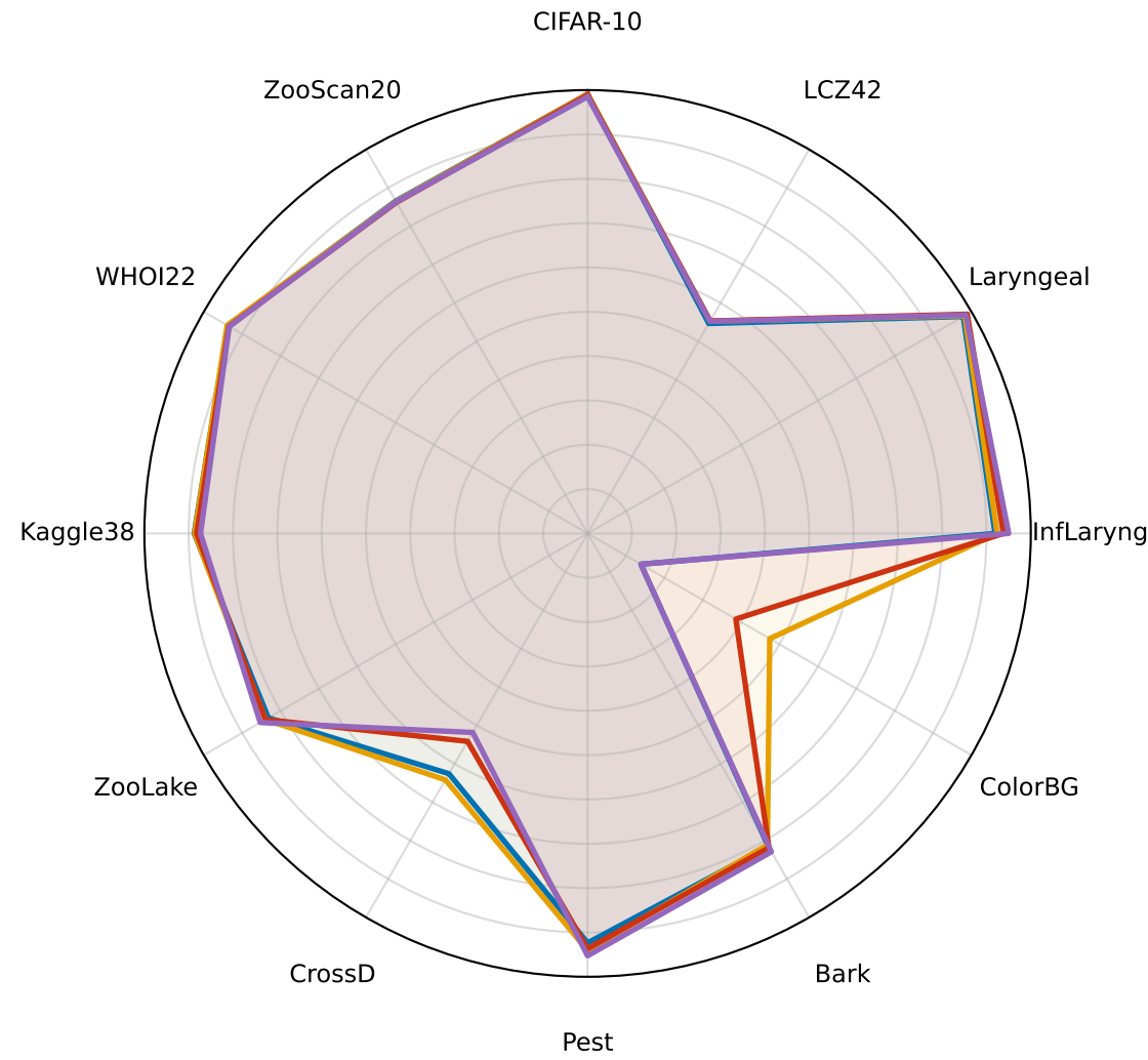
DINOv2
