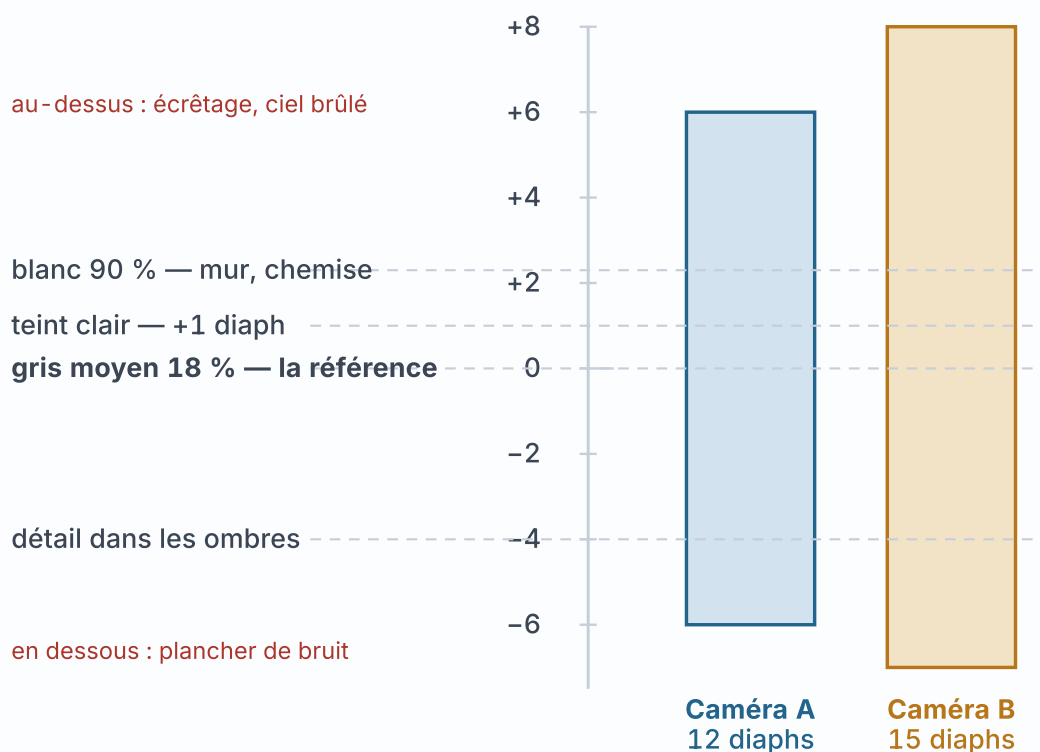
Fig. 21.3 L'échelle est calée sur le gris moyen. La caméra B ne donne pas automatiquement « une plus belle image » — elle vous donne de la marge : un ciel non brûlé derrière le comédien et des ombres qui gardent du détail. Concrètement, chaque diaph supplémentaire au-dessus du gris moyen est une fenêtre sauvée dans la pièce.
