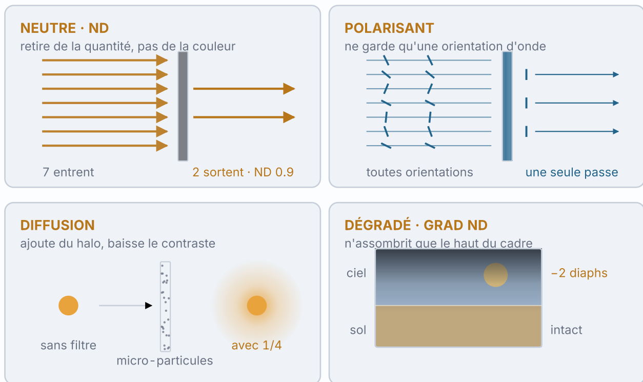
Fig. 29.1 Les quatre familles, et ce que chacune retire ou ajoute au faisceau. Le neutre (ND) retire de la quantité sans toucher à la couleur : il rend le grand diaphragme possible en plein soleil. Le polarisant ne retire qu'une orientation d'onde : les reflets du verre, de l'eau et du feuillage disparaissent, le ciel fonce. La diffusion disperse une part de la lumière autour des hautes lumières : les halos apparaissent, le contraste baisse, la peau s'adoucit. Le dégradé ne travaille que sur la moitié haute du cadre : il rattrape un ciel de trois diaphragmes trop clair.
