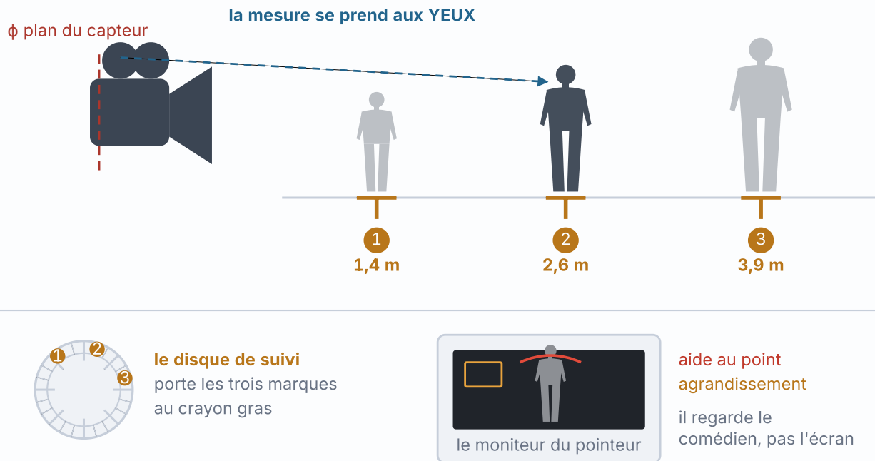
Fig. 30.2 L'organisation du poste. Le disque du suivi de point porte les marques au crayon ; la mesure se prend du plan du capteur — sigle \phi sur le flanc de la caméra — aux yeux du comédien ; le moniteur du pointeur affiche l'aide au point ( focus peaking ) et l'agrandissement. Sur le trajet en trois temps représenté ici, chaque arrêt a sa marque au sol et sa graduation correspondante sur le disque.
