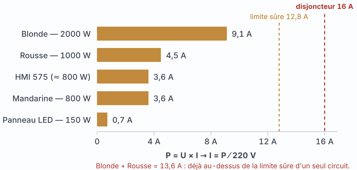
Fig. 26.1 Le réseau marocain est en 220 volts / 50 Hz, et le disjoncteur domestique habituel est de 16 A. La règle professionnelle : ne dépassez pas 80 % du disjoncteur (12,8 A ≈ 2800 W), parce que les lampes tungstène appellent un courant bien plus élevé au premier instant (courant d'appel) et font sauter le disjoncteur à l'allumage plutôt qu'en fonctionnement.
