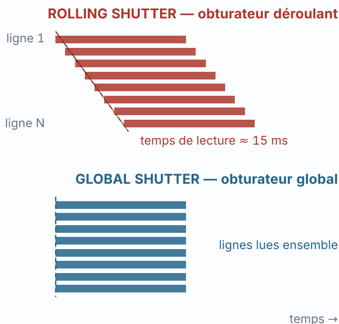
Fig. 21.2 Les barres représentent l'instant de lecture de chaque ligne. En rolling shutter, les lignes du bas ont 10 à 25 millisecondes de retard sur celles du haut : tout ce qui est vertical penche pendant un panoramique rapide, le flash se coupe en deux, l'image gélatine dans les plans d'hélicoptère. Le global shutter règle le problème mais coûte un diaph ou plus de plage dynamique.
