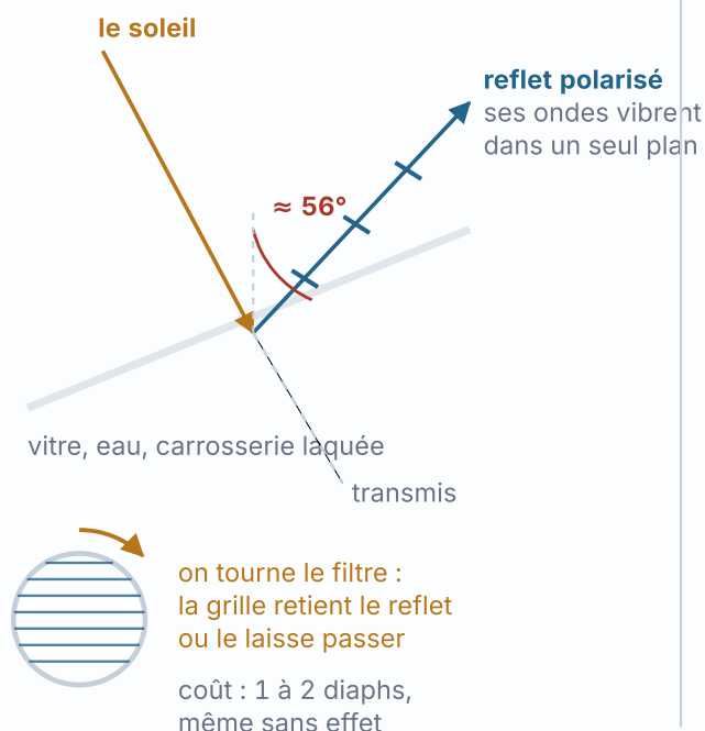
Fig. 29.2 À gauche, la mécanique : la lumière directe vibre dans toutes les directions, celle que la vitre renvoie est polarisée — ses ondes vibrent dans un seul plan —, et la grille du filtre la retient ou la laisse passer selon l'orientation qu'on lui donne. L'effet est maximal quand la surface est vue vers 56° . À droite, la même chose vue de dessus, pour le ciel : le maximum se produit dans la bande à 90° du soleil , et l'on n'obtient rien du tout en visant le soleil ou en lui tournant le dos — c'est pourquoi un panoramique polarisé fait respirer le bleu du ciel de façon très visible, puis l'aplatit.
