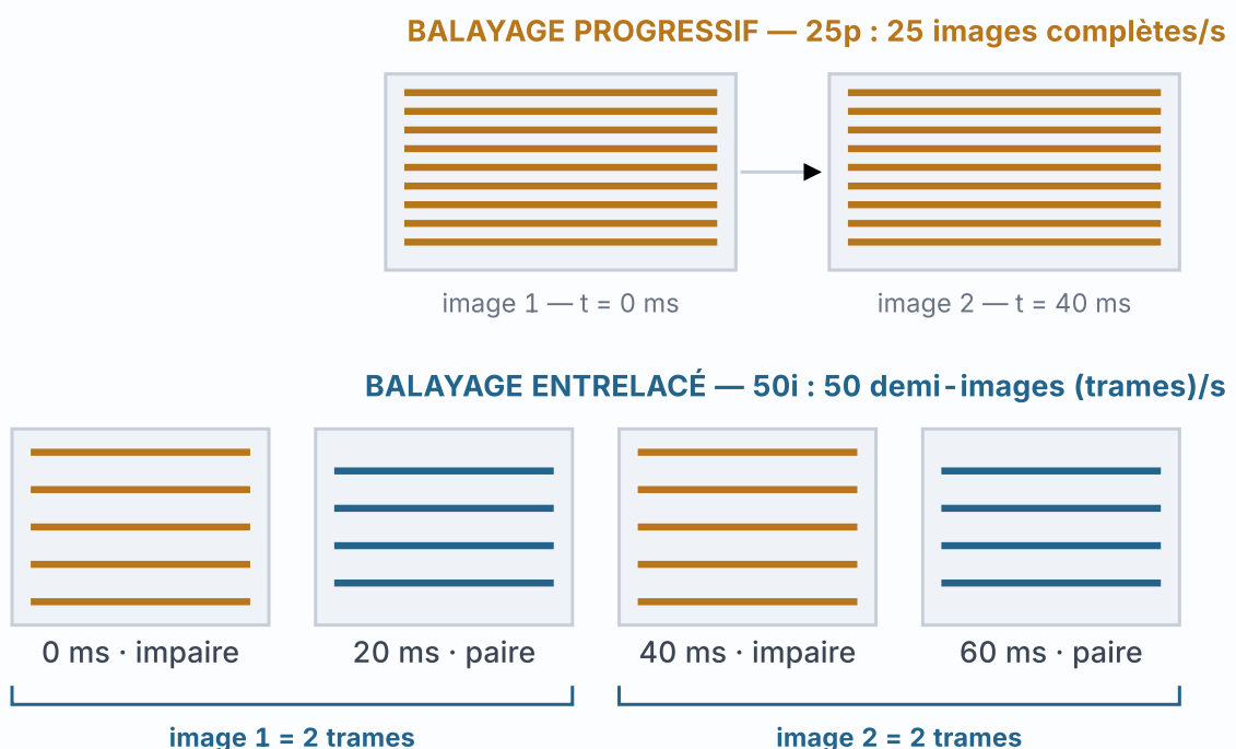
Fig. 27.1 En progressif, chaque image est complète et prise en un seul instant. En entrelacé, les lignes impaires sont lues d'abord, les paires 20 millisecondes plus tard, et les deux trames sont fusionnées en une seule « image ». C'est pourquoi, si quelque chose bouge entre les deux trames, des dents de peigne apparaissent sur ses contours : c'est le peignage .
