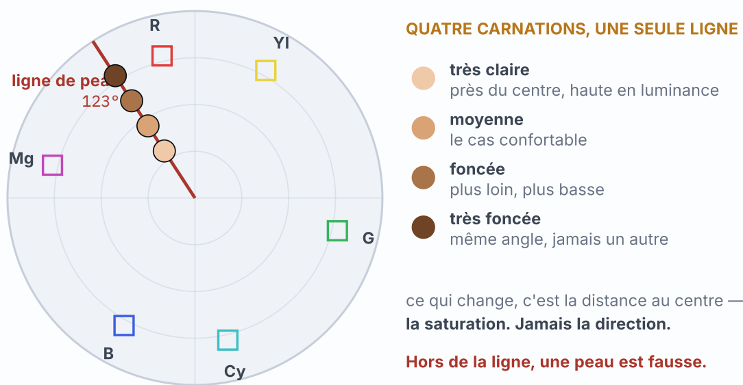
Fig. 30.1 Le vectorscope et sa ligne de peau (skin tone line, I-line), à 123° environ. Quatre carnations, de la plus claire à la plus foncée, se posent toutes sur cette ligne : ce qui change entre elles, c'est la distance au centre — la saturation — et la luminance, presque jamais l'angle. Une peau qui quitte la ligne est une peau fausse.
