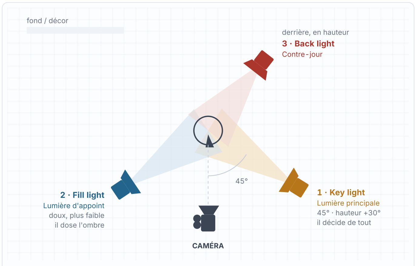
Fig. 20.1 Vue de dessus. Les 45° entre l'axe caméra et la lumière principale sont la valeur de référence : assez pour créer du volume sur le visage sans en noyer la moitié dans le noir.
