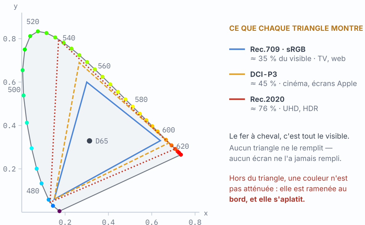
Fig. 31.1 Le fer à cheval du CIE 1931 : tout ce que l'œil humain peut voir. À l'intérieur, trois triangles emboîtés — Rec.709, DCI-P3, Rec.2020 — et le point blanc D65 qui leur sert de repère commun. Aucun triangle ne couvre le fer à cheval entier : aucun écran n'a jamais montré toutes les couleurs que vous voyez.
