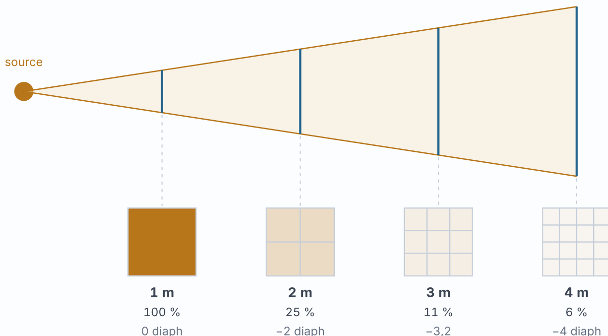
Fig. 18.1 La même quantité de lumière se répartit sur un carré à un mètre, sur 4 carrés à deux mètres, sur 16 à quatre mètres. Chaque carré en reçoit une part plus petite : c'est le 1/d^2 .
