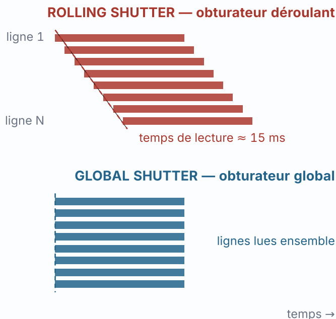
Fig. 33.2 Les barres représentent l'instant de lecture de chaque ligne. En rolling shutter, les lignes du bas ont 10 à 25 millisecondes de retard sur celles du haut : tout ce qui est vertical penche pendant un panoramique rapide, le flash se coupe en deux, l'image gélatine dans les plans d'hélicoptère. Le global shutter règle le problème mais coûte un diaph ou plus de plage dynamique.
