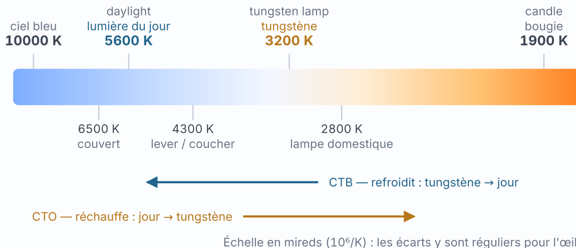
Fig. 19.1 L'échelle est graduée en mireds et non directement en kelvins, parce que l'écart entre 3200 et 3400 se voit à l'œil alors que celui entre 9000 et 9200 ne se voit presque pas. Les gélâtines CTO et CTB déplacent la source sur cette échelle.
