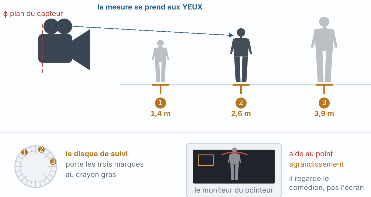
Fig. 48.2 L'organisation du poste. Le disque du suivi de point porte les marques au crayon ; la mesure se prend du plan du capteur — sigle \phi sur le flanc de la caméra — aux yeux du comédien ; le moniteur du pointeur affiche l'aide au point ( focus peaking ) et l'agrandissement. Sur le trajet en trois temps représenté ici, chaque arrêt a sa marque au sol et sa graduation correspondante sur le disque.
