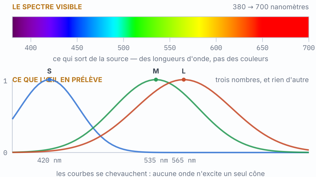
Fig. 25.1 En haut, le spectre visible : de 380 nm (violet) à 700 nm (rouge). En dessous, les trois cônes de l'œil ( S, M, L cones ) et ce qu'ils captent. Remarquez que leurs courbes se chevauchent largement : aucune longueur d'onde n'excite un seul cône. C'est de ce chevauchement que naît toute la colorimétrie — et le métamérisme avec.
