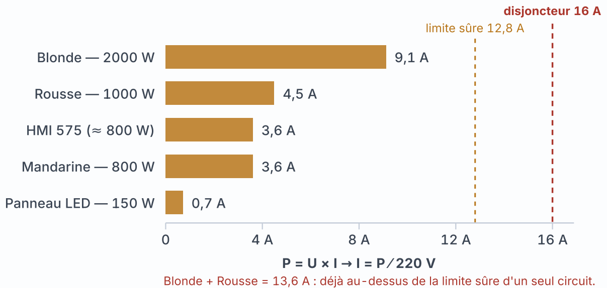
Fig. 38.1 Le réseau marocain est en 220 volts / 50 Hz, et le disjoncteur domestique habituel est de 16 A. La règle professionnelle : ne dépassez pas 80 % du disjoncteur (12,8 A ≈ 2800 W), parce que les lampes tungstène appellent un courant bien plus élevé au premier instant (courant d'appel) et font sauter le disjoncteur à l'allumage plutôt qu'en fonctionnement.
