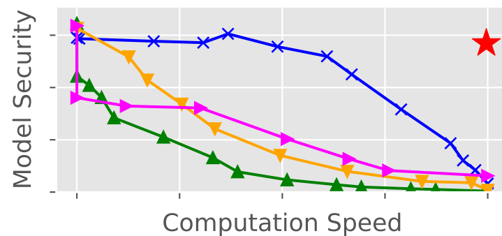
VGG16_BN
