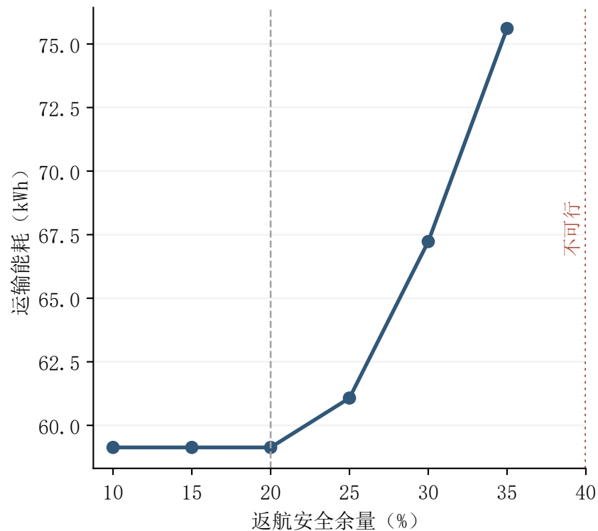
安全余量敏感性：每个情景均重新优化组批
