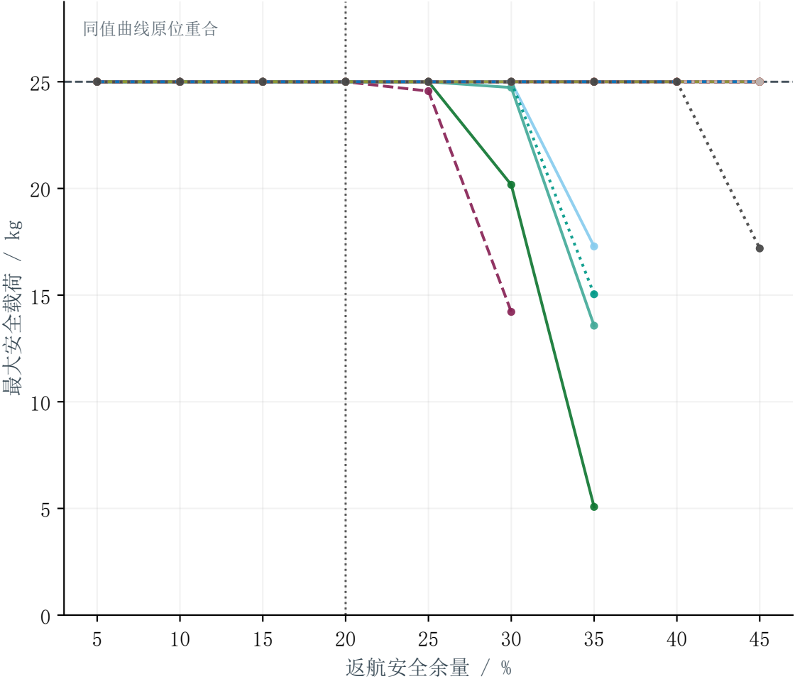
A型 • 额定载质量 25 kg
