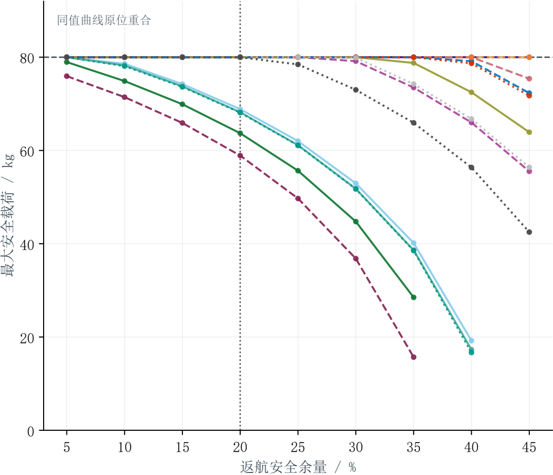
C型 • 额定载质量 80 kg
