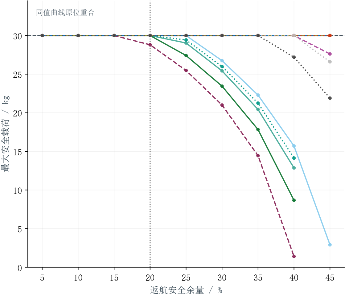
B型 • 额定载质量 30 kg
