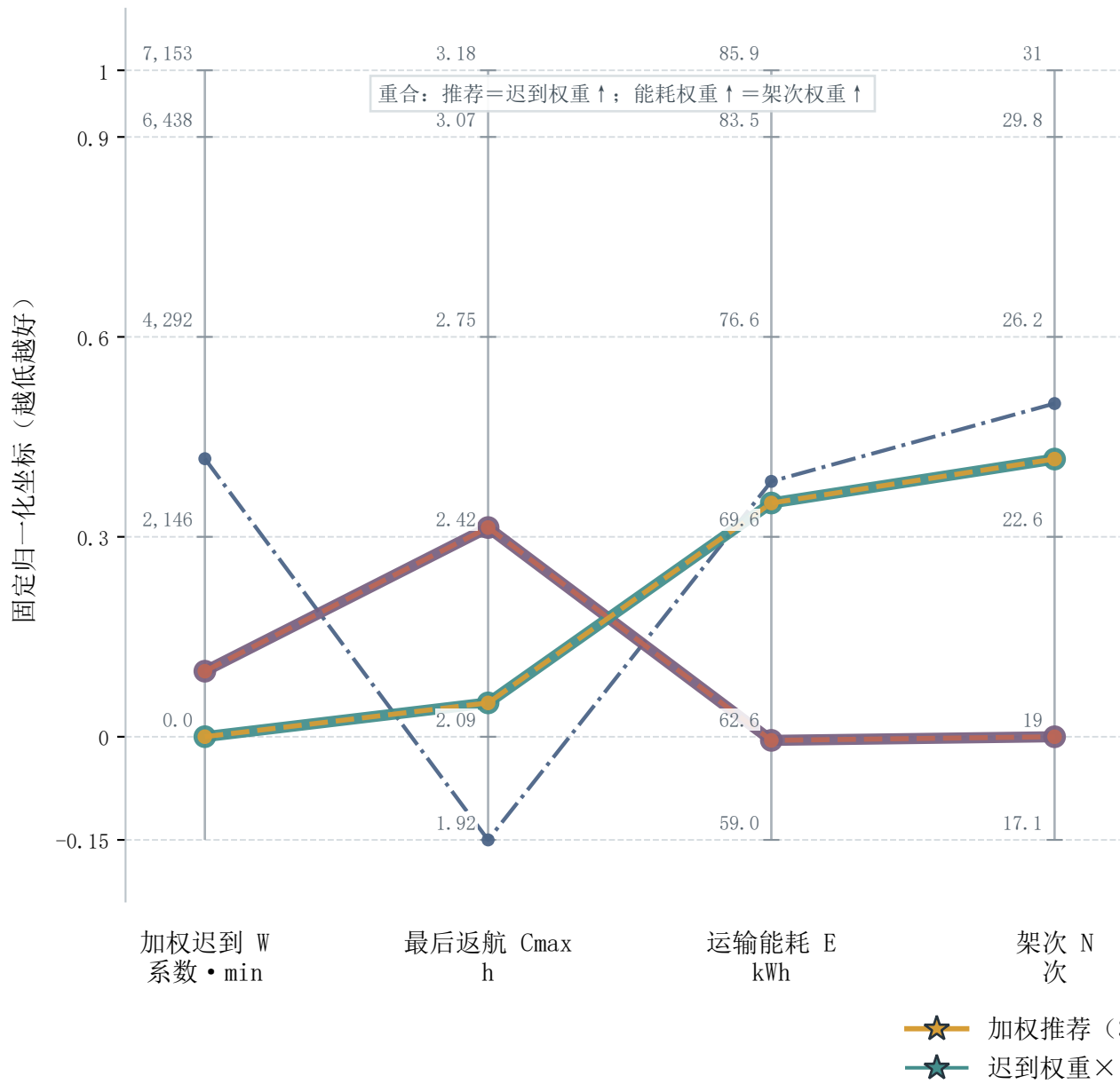
(a) 五方案平行坐标：各轴刻度标实际值
