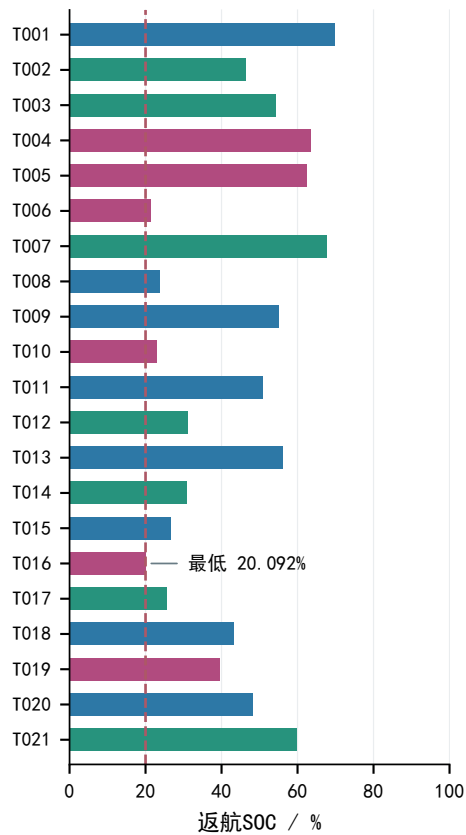
(b) 运输返航安全余量
