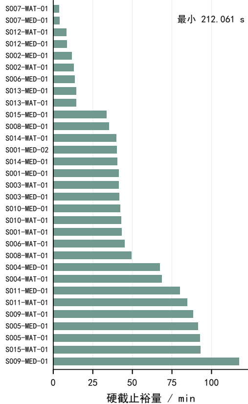
(a) 31箱硬截止裕量
