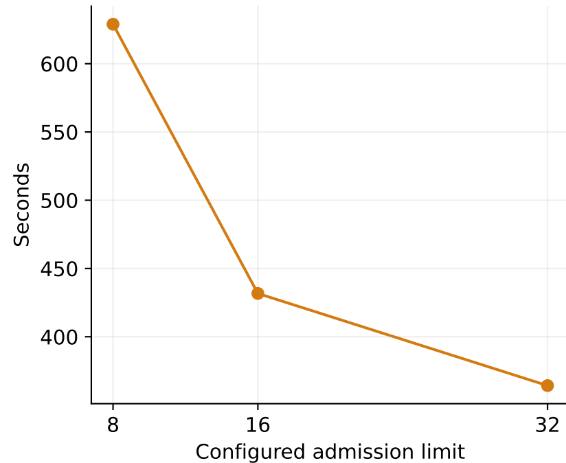
P99 TTFT
