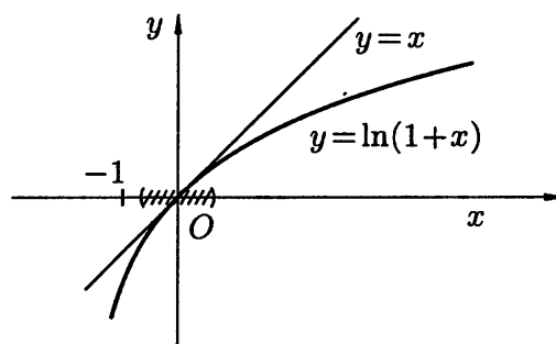
Рис. 116. \ln(1+x) \approx x \quad (x \rightarrow 0)
