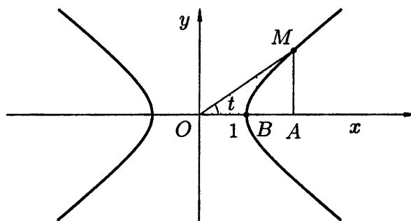
Рис. 137. Параметрические уравнения x = \operatorname{ch} t и y = \operatorname{sh} t определяют гиперболу x^2 - y^2 = 1 , причем OA = \operatorname{ch} t , AM = \operatorname{sh} t
