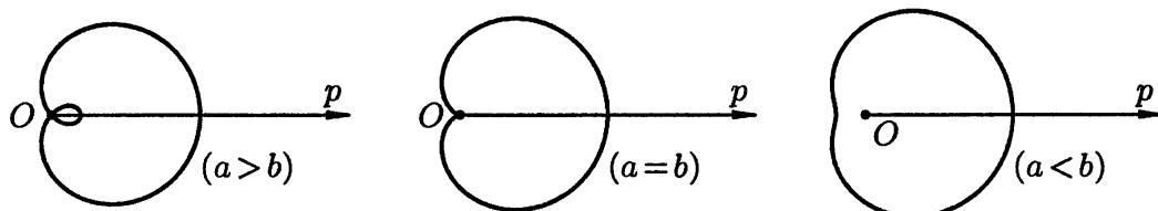
Рис. 35. Улитка Паскаля
