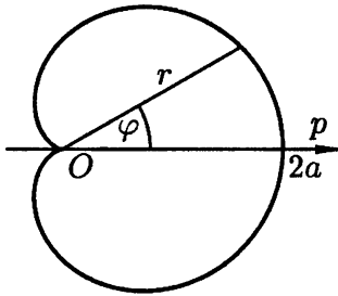
Рис. 38. Кардиоида Уравнение в полярных координатах имеет вид r = a(1 + \cos \varphi) , где a > 0 . Кардиоида — частный случай улитки Паскаля ( a = b ).
