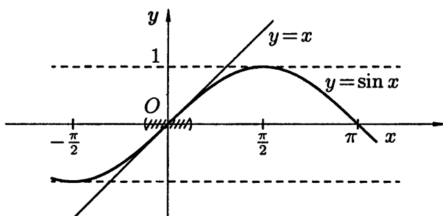
Рис. 115. \sin x \approx x \quad (x \rightarrow 0)
