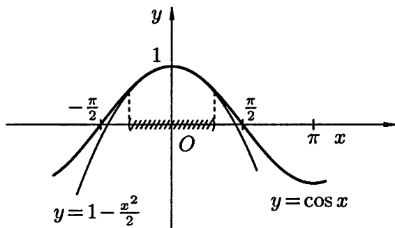
Рис. 117. \cos x \approx 1 - \frac{x^2}{2} ( x \rightarrow 0 )
