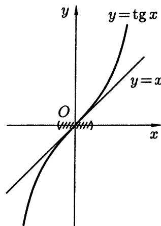
Рис. 114. \operatorname{tg} x \approx x \quad (x \rightarrow 0)
