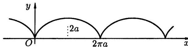
Рис. 40. Циклоида
