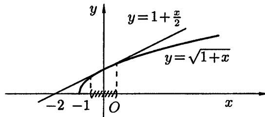
Рис. 118. \sqrt{1+x} \approx 1 + \frac{x}{2} ( x \rightarrow 0 )
