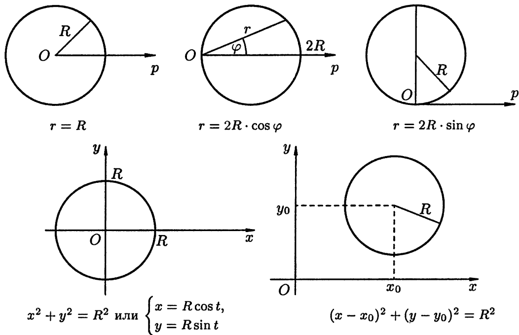
Рис. 32. Окружность радиуса R
