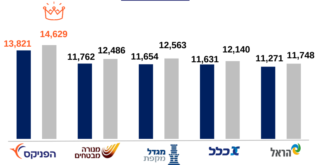
שכר ממוצע ₪
