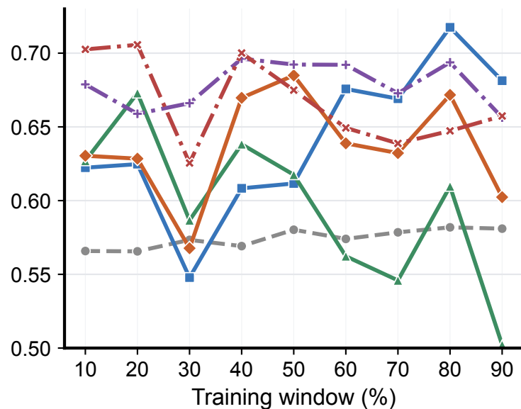
F1
