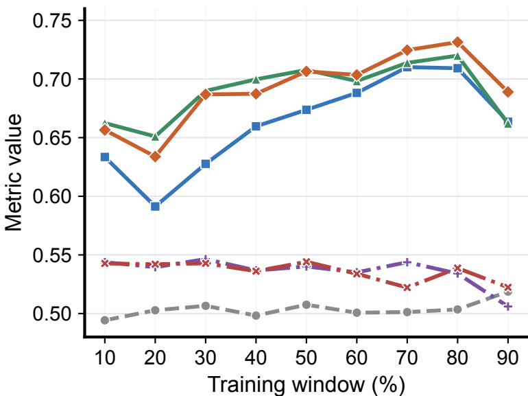
AUC
