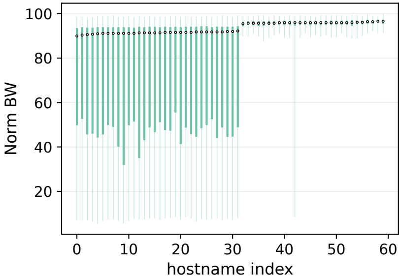
nvlink-only AllGather
