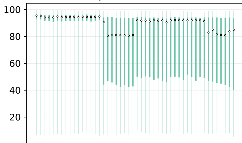
nvlink-only AllGather 8r/1n 18 MiB
