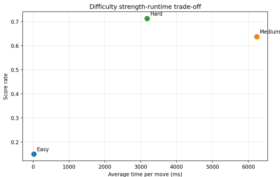
FIGURE 8 – Compromis entre la force de jeu et le temps moyen de calcul par coup.
