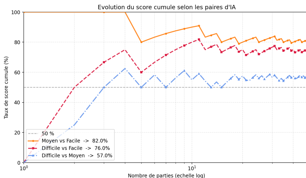
FIGURE 4 – Évolution du score cumulé pour la sélection théorique A1/B2/B3.
