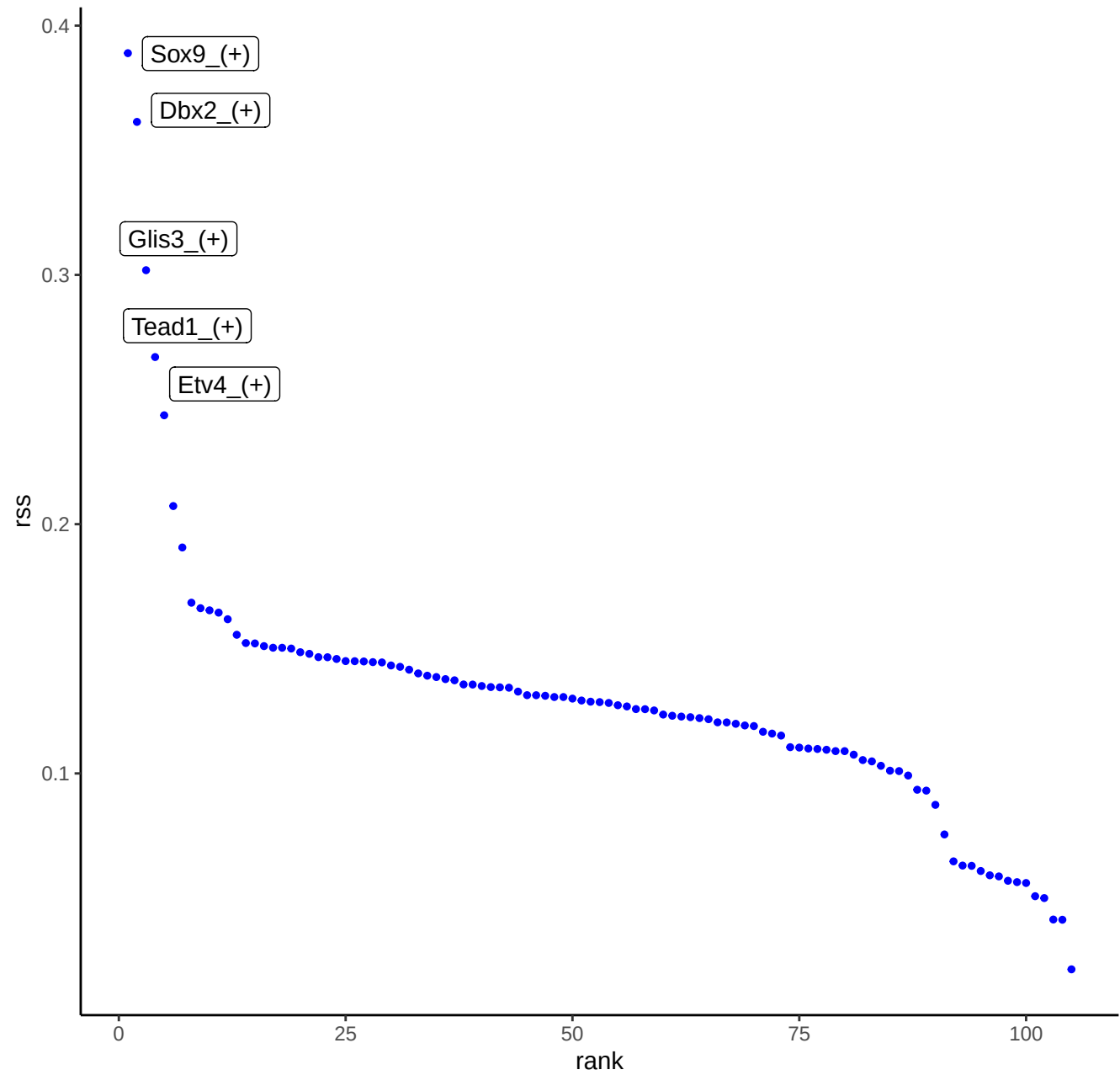
Astro1
