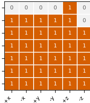
MACE-POLAR-1
