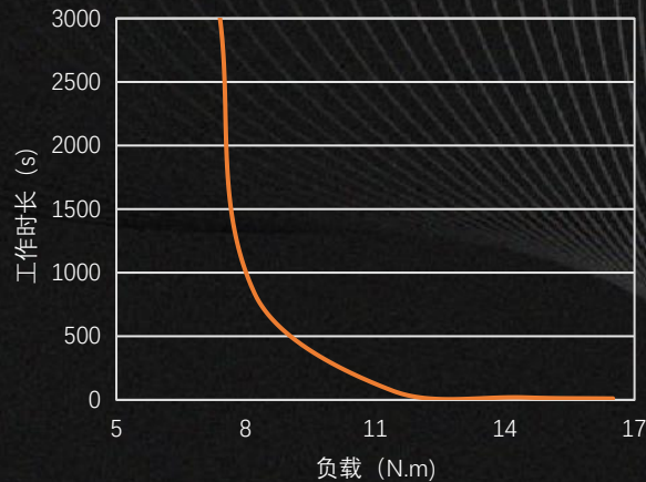
堵转工况最大过载曲线 (Max Overload)
