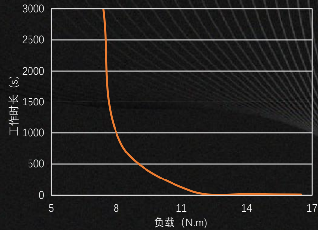
旋转工况最大过载曲线 (Max Overload) (150mm×150mm铝散热板)
