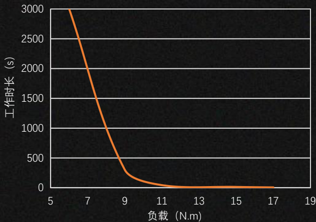
堵转工况最大过载曲线 (Max Overload)
