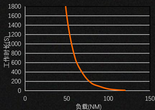
堵转工况最大过载曲线 (Max Overload)
