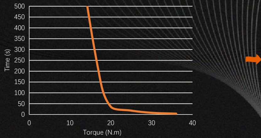
堵转工况最大过载曲线 (Max Overload)
