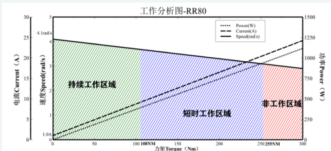
性能曲线图
