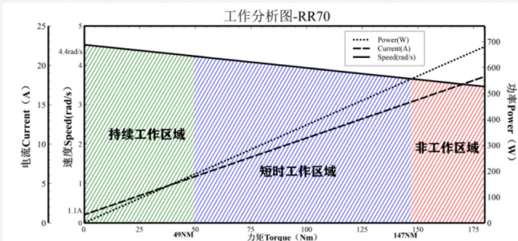
性能曲线图
