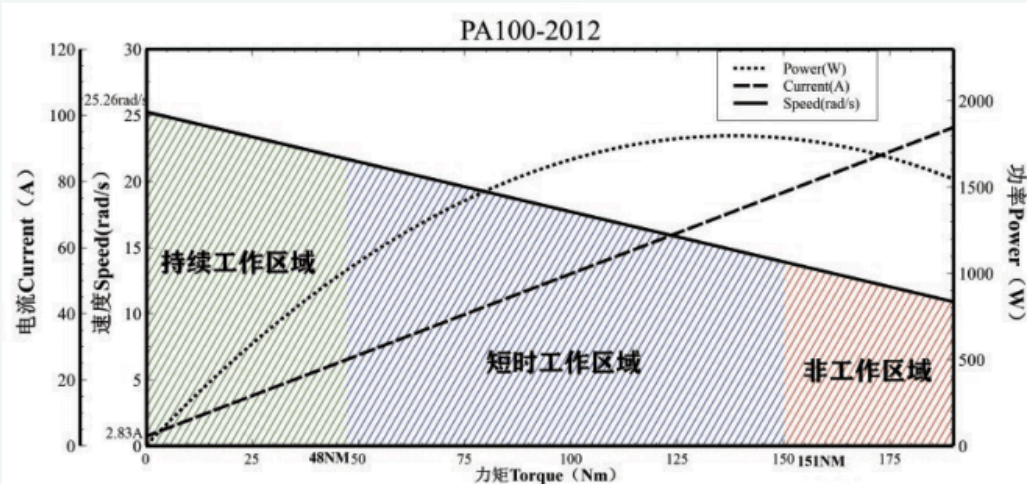
性能曲线图
