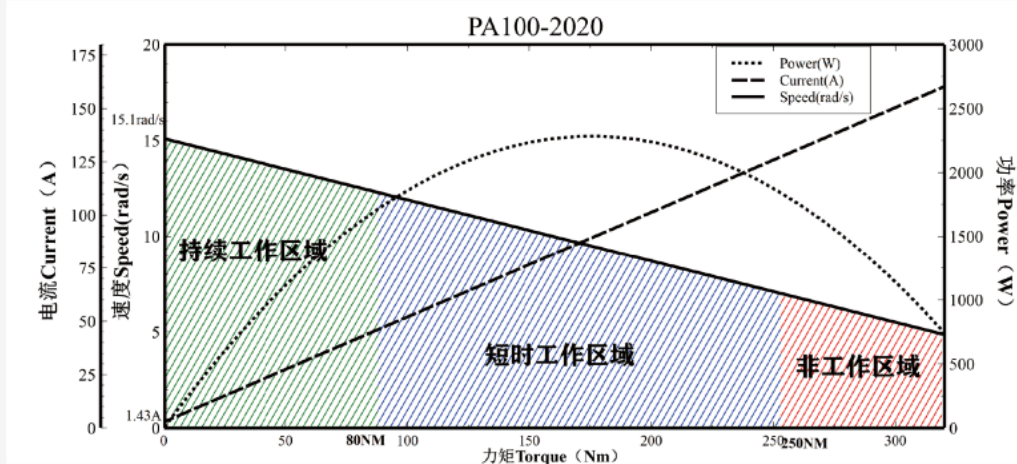
性能曲线图
