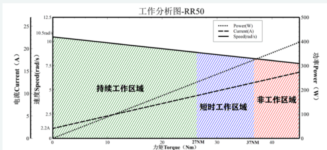
性能曲线图
