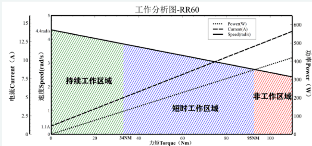
性能曲线图
