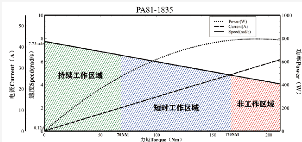
性能曲线图
