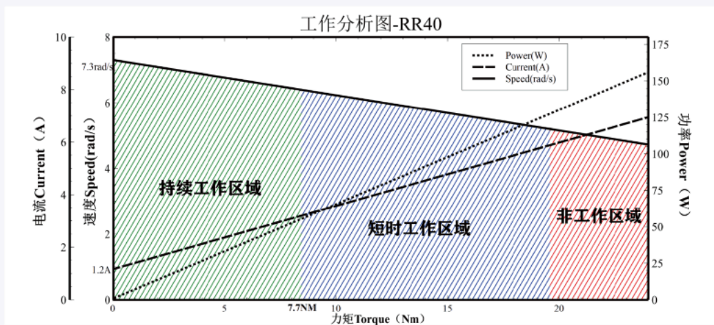
性能曲线图
