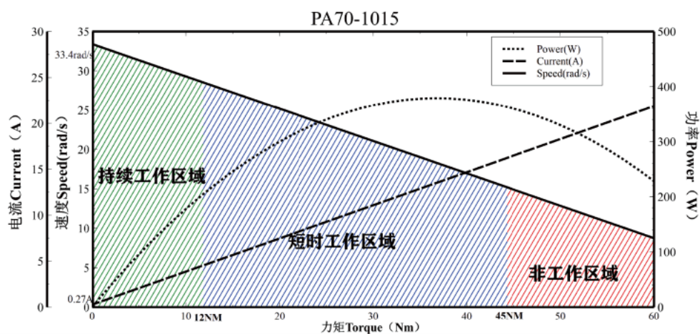
性能曲线图
