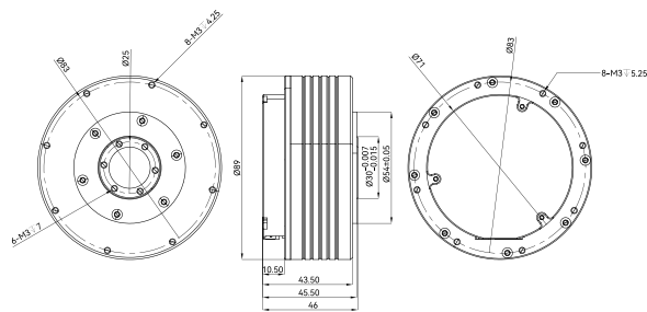
产品图纸
