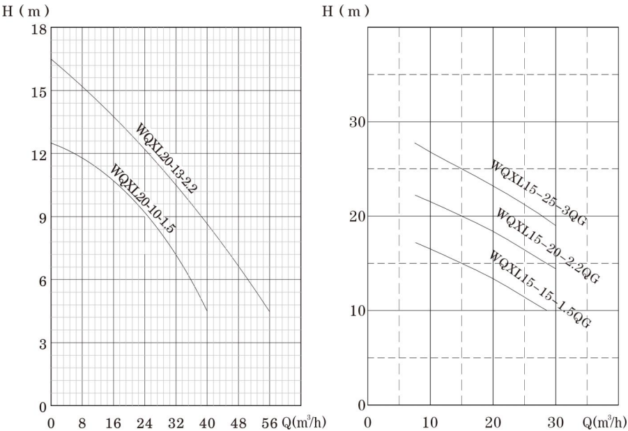
性能曲线图
