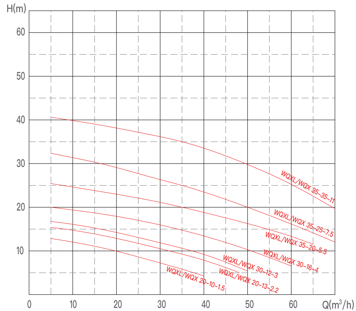
旋流泵
