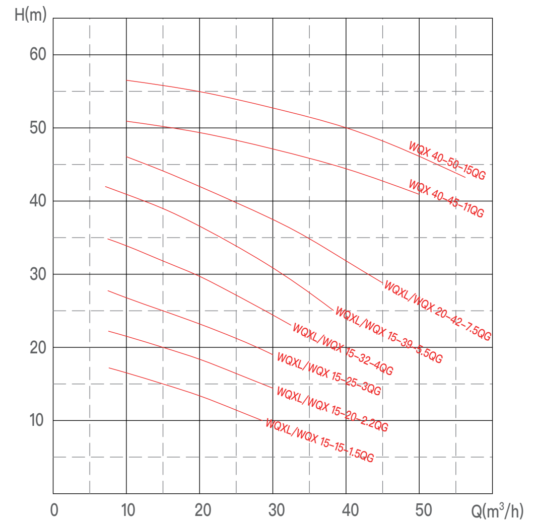
切割泵
