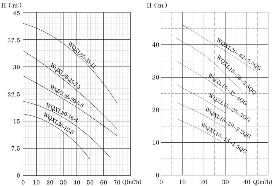
性能曲线图
