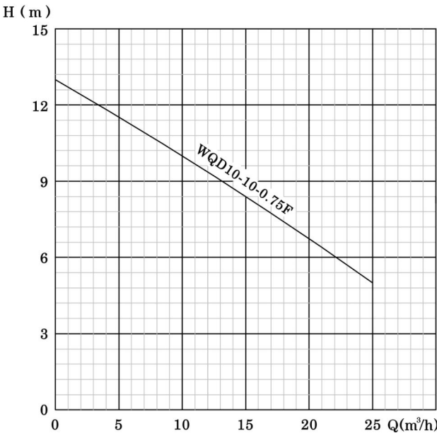
性能曲线图
