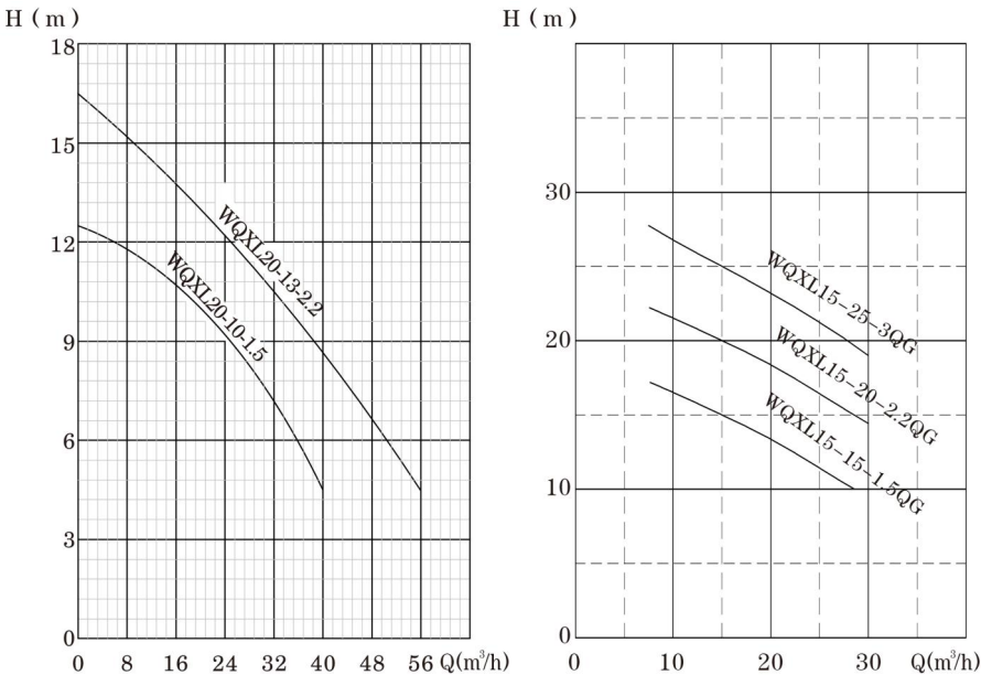
性能曲线图
