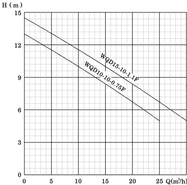
性能曲线图
