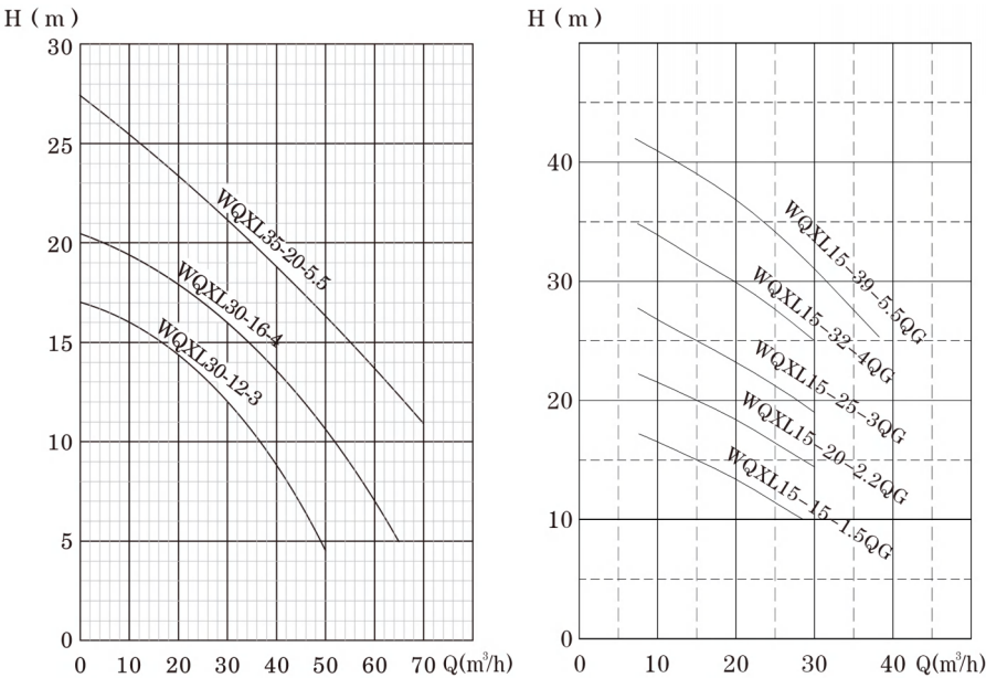
性能曲线图
