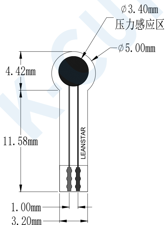
SI4-G 柔性薄膜压力传感器尺寸图
