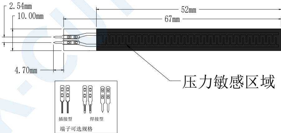
ZD10-100 柔性压力传感器尺寸图
