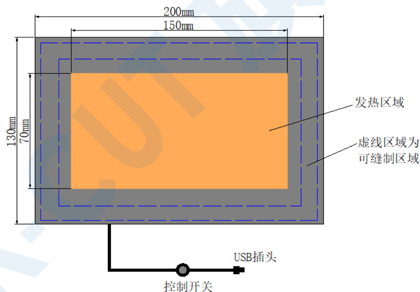
图1 发热片结构及尺寸图
