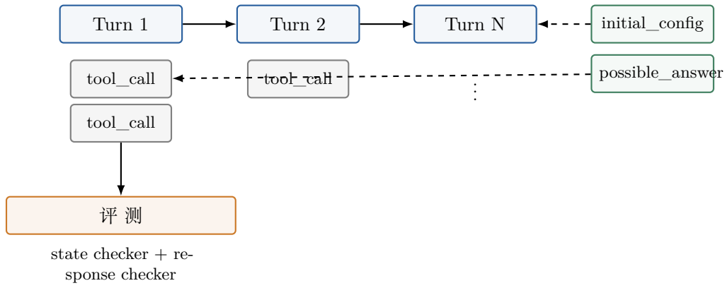
图 4: BFCL 多轮任务结构。每个用户轮次可包含多个工具调用步骤, possible_answer 提供逐轮参考调用, 评测同时检查状态和调用路径。
