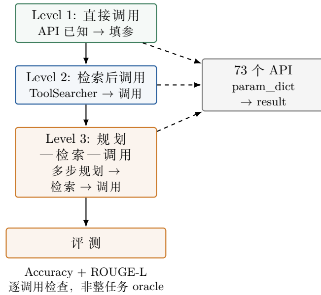
图 5: API-Bank 三级任务结构。从直接调用到检索后调用再到规划多步调用，难度递进。评测按逐调用一致性检查，不提供整对话最终状态 oracle。
