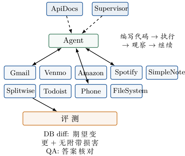
图 6: AppWorld 任务结构。Agent 在 9 个应用和 2 个辅助应用组成的沙盒中，通过编写代码—执行—观察循环完成跨应用任务，评测基于数据库 diff 的程序化测试。
