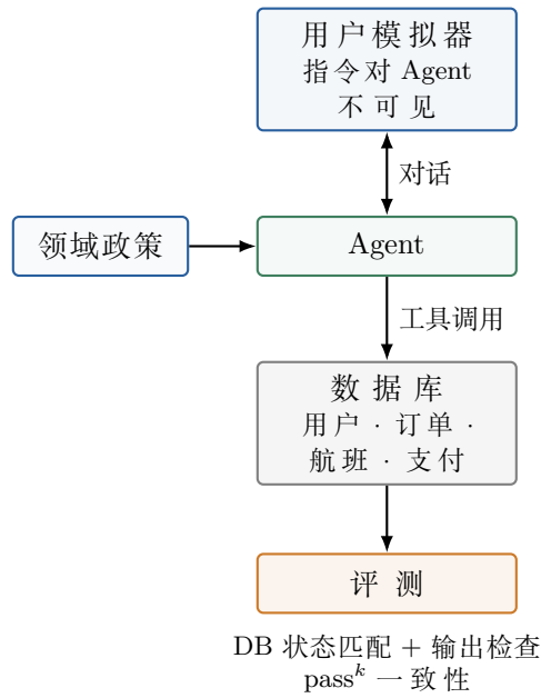
图 3: \tau -bench 任务结构。Agent 与用户模拟器对话，调用数据库工具完成客服任务，评测比较最终数据库状态和回复内容。
