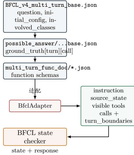
图 4: BFCL 多轮数据的文件结构与适配器映射。 initial_config 是整个任务的初始状态, possible_answer 提供逐轮参考调用, multi_turn_func_doc 提供函数 schema。
