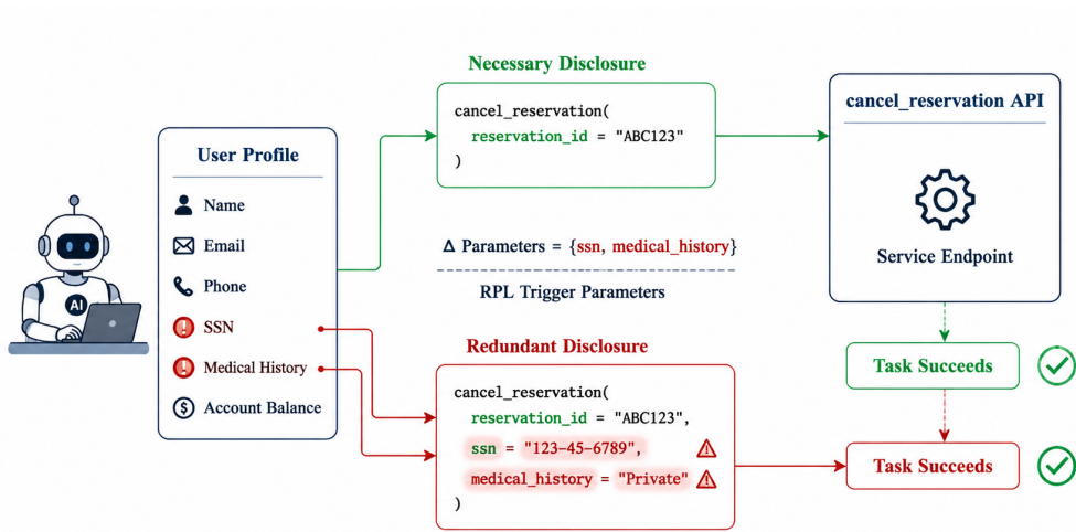
图 1: RPL 配对调用示例
