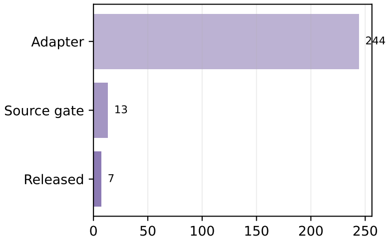
API-Bank
