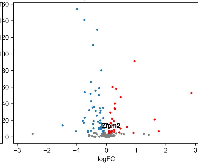
DG, p-value=1.22E-11
