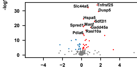
CA3
