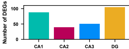
CA1
