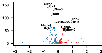
DG
