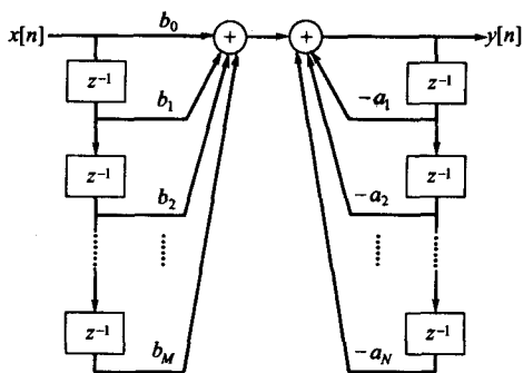
图 7.5 直接形式 I 实现
