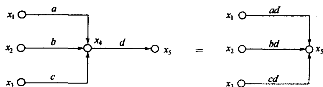
(a) 混合极点的消除
