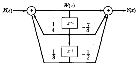
图 7.15 例 7.33 直接 II 型
