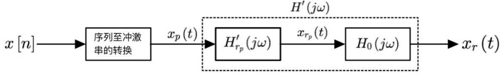
图 3-1 采用离散预校正的零阶保持恢复系统（等效模型）
