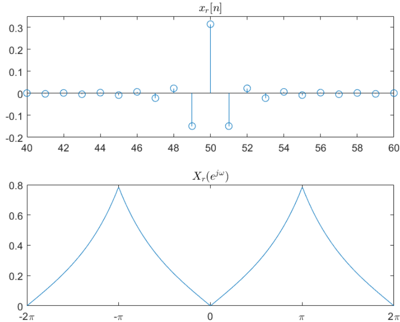
图 3-4 校正后的离散时间序列 x_r[n] 及其频谱 X_r(e^{j\omega})
