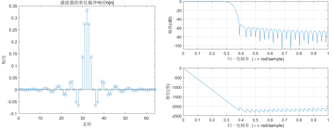
图 3-6 用海明窗设计的 FIR 滤波器特性
