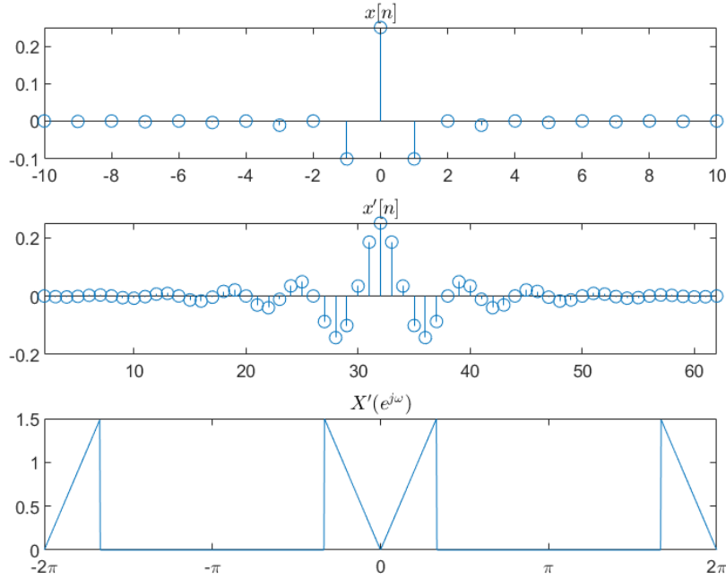
图 3-7 内插后的序列 x'[n] 及其频谱 X'(e^{j\omega})
