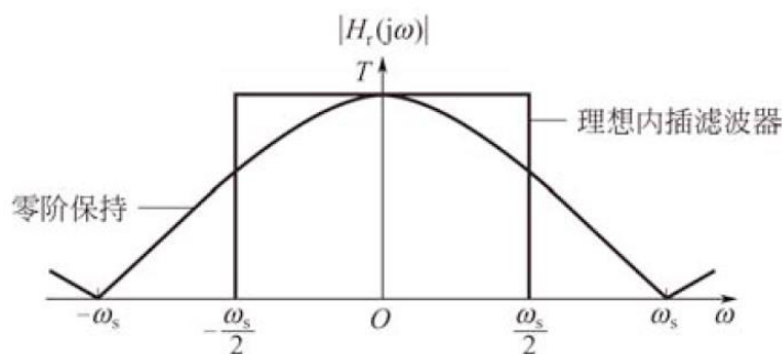
图 1-2 零阶保持和理想滤波器的频响特性
