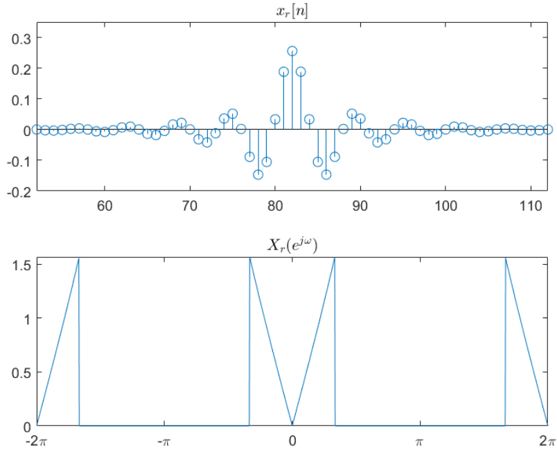
图 3-8 离散预校正后得到的 x_r[n] 及其频谱 X_r(e^{j\omega})
