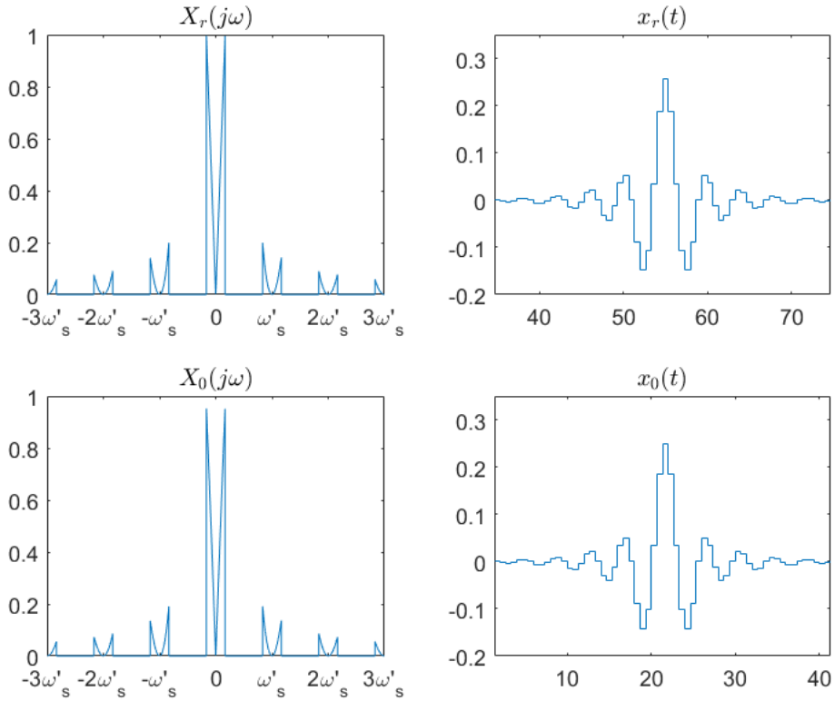
图 3-9 x_r(t) , x_0(t) 及其频谱对比
