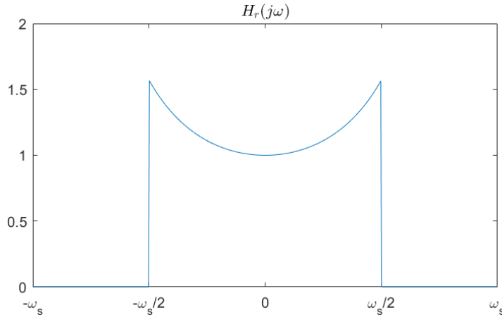
图 2-2 H_r(j\omega) 的频率响应特性
