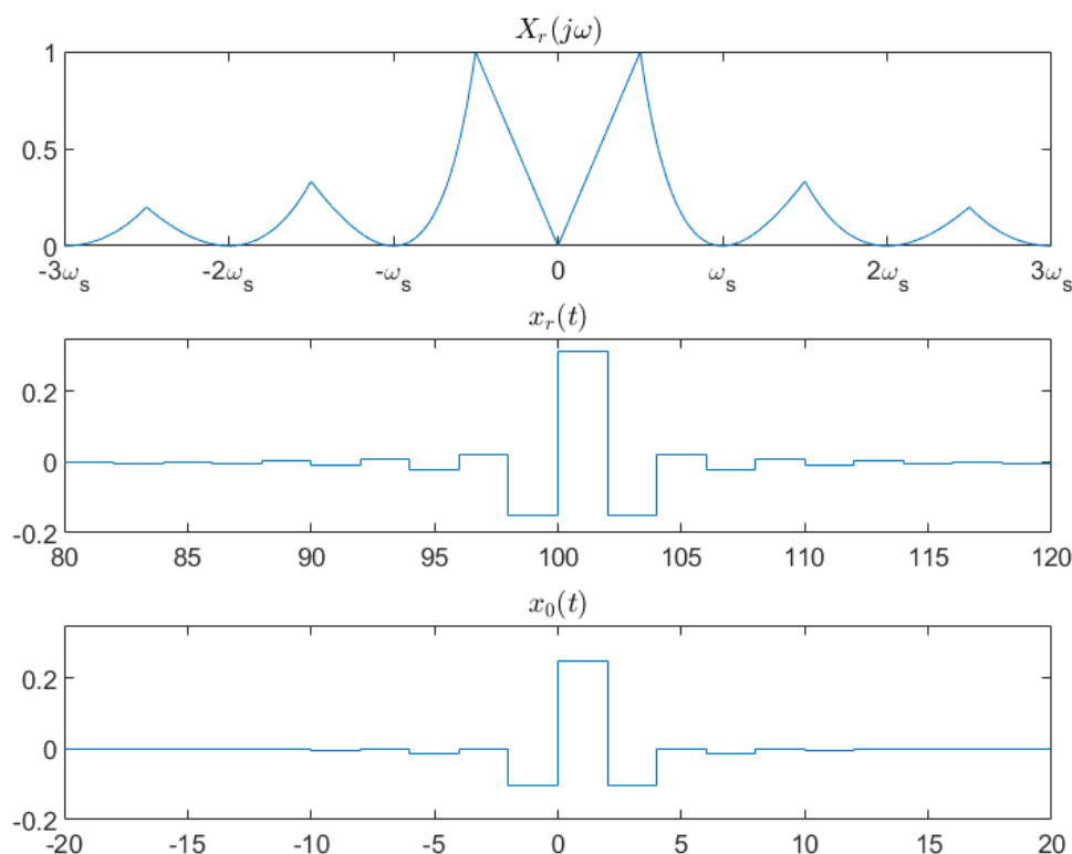
图 3-5 重建信号 x_r(t) 及其频谱 X_r(j\omega)
