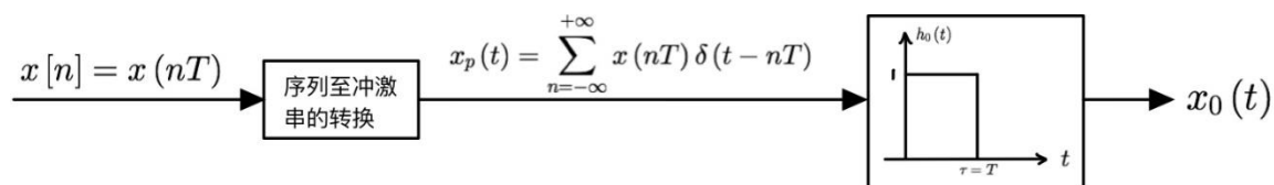
图 1-1 零阶保持系统
