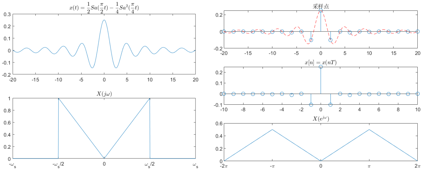
图 3-3 原始信号 x(t) 和样值序列 x[n]
