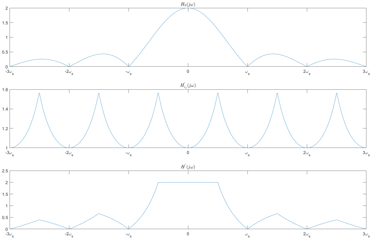
图 3-2 整个重建系统的频率响应 H'(j\omega)
