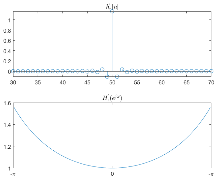
图 3-1 离散预校正系统的单位脉冲响应和频响特性
