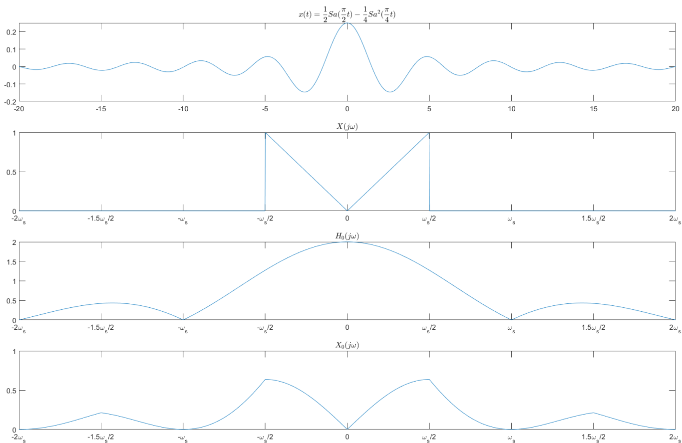
图 1-3：零阶保持系统频谱失真验证实验
