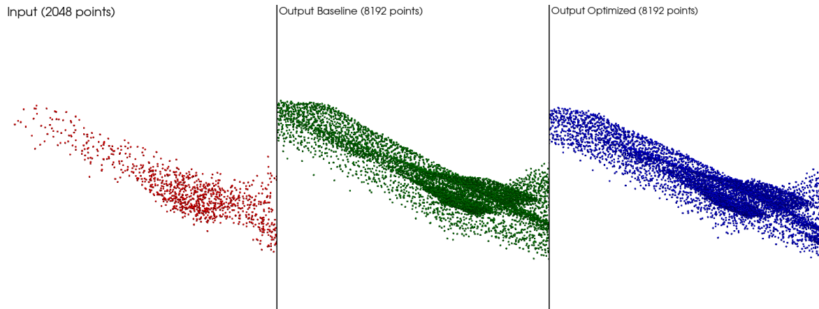
图 4.3 飞机残缺区域补全密度细节对比
