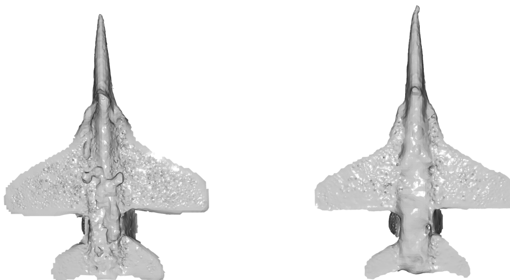
图 4.8 飞机网格重建结果仰视视图对比（左：PoinTr 基线，右：本算法优化）
