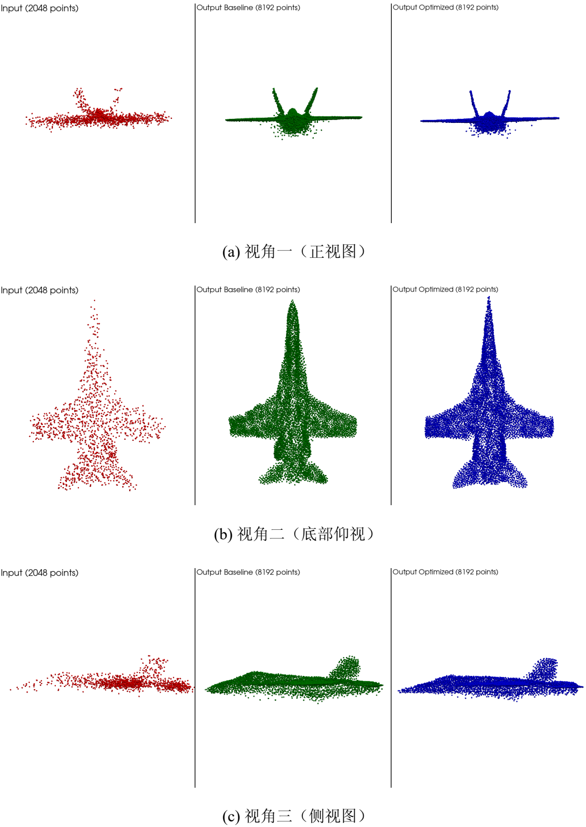
图 4.2 飞机补全效果对比
