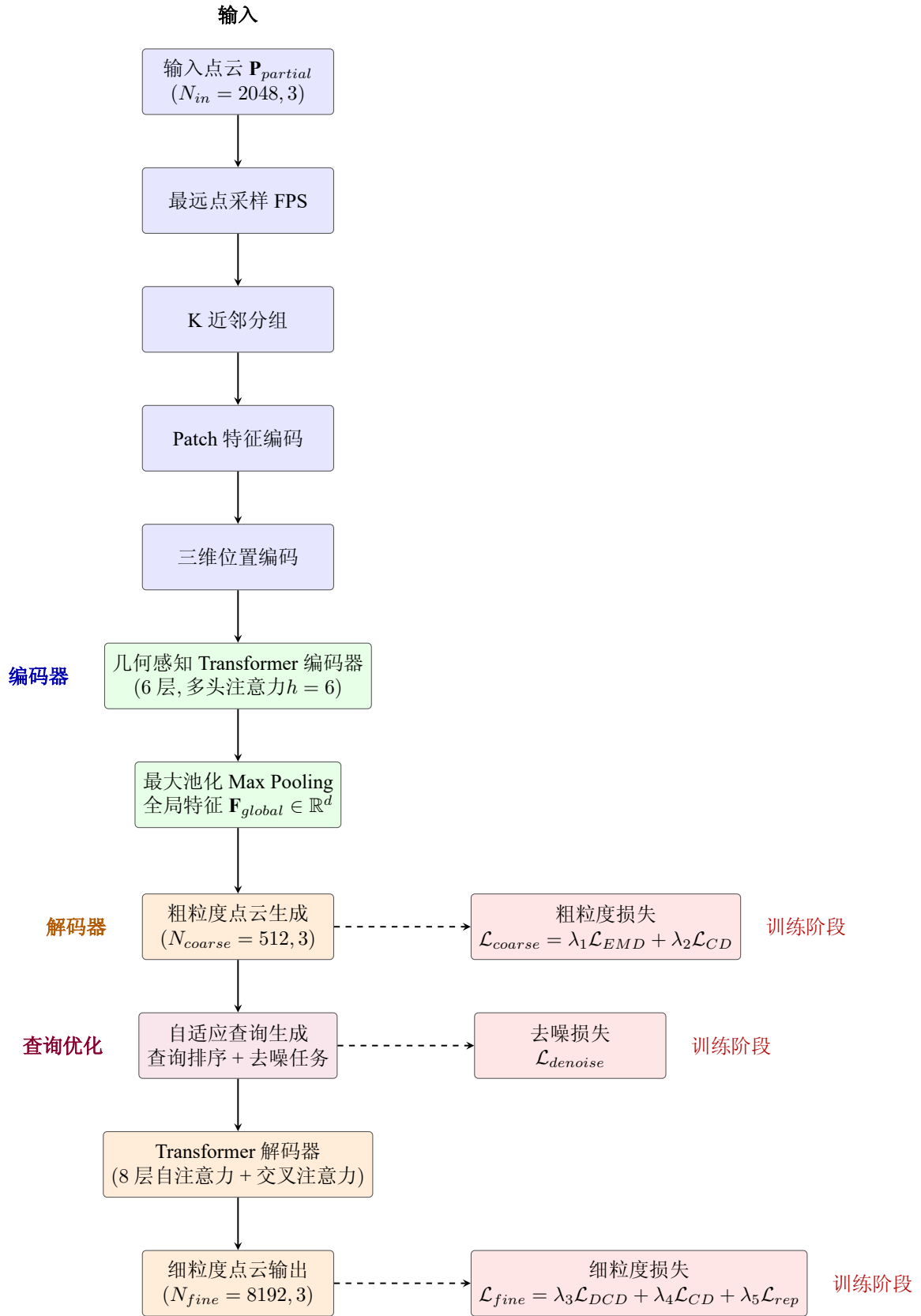
图 3.1 基于 Transformer 的点云补全网络整体架构图
