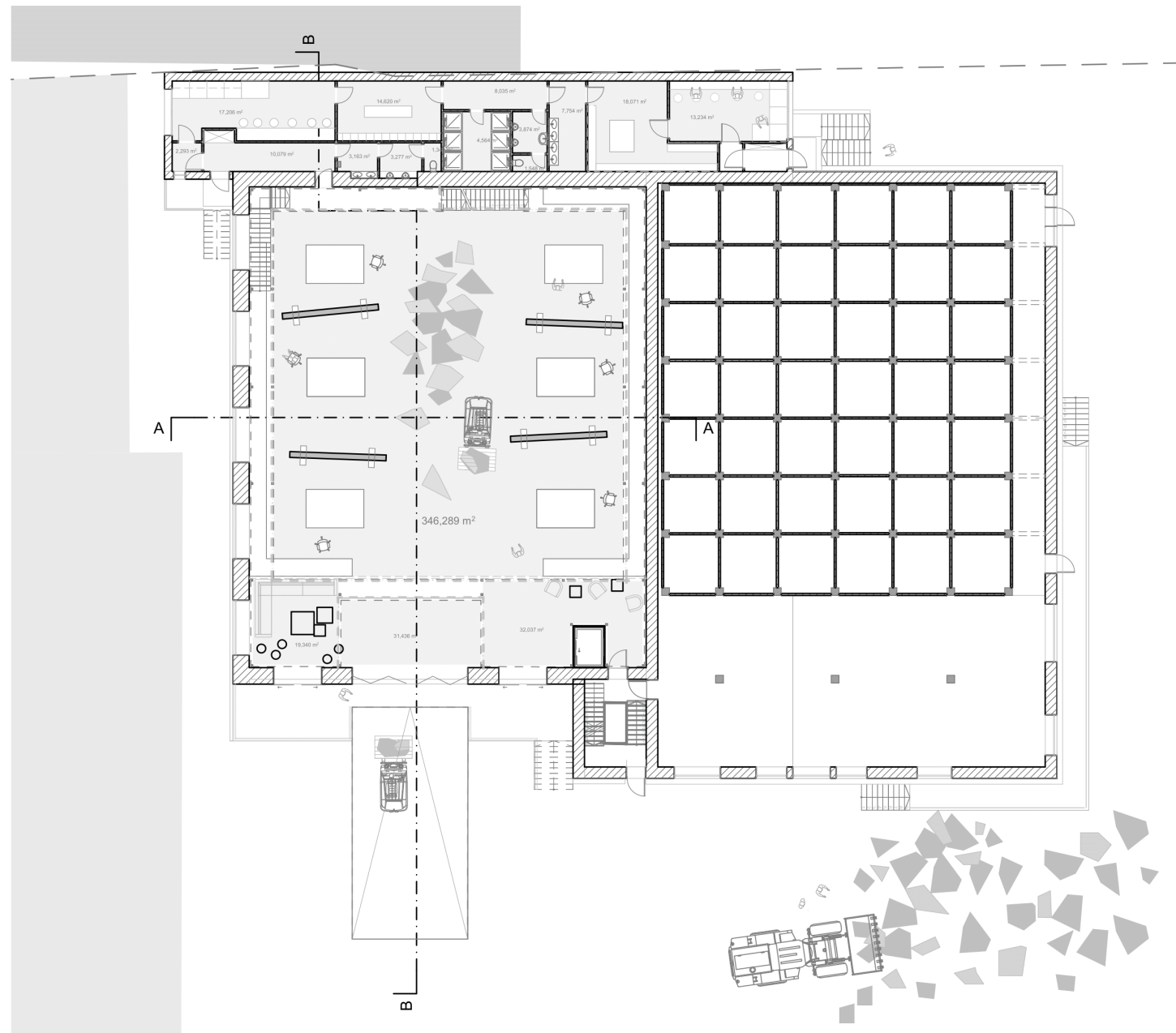
MH2 - vázlatterv - Gelencsér György Karsa – Muzsai Nimród – fsz alaprajz 1:200– 2025.11.24
