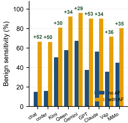
A AF ablation (9 models)
