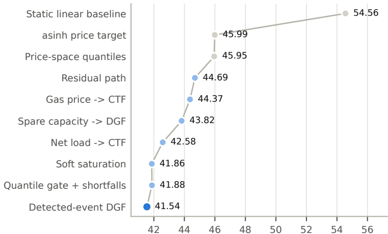
Test MAE (AUD/MWh)
