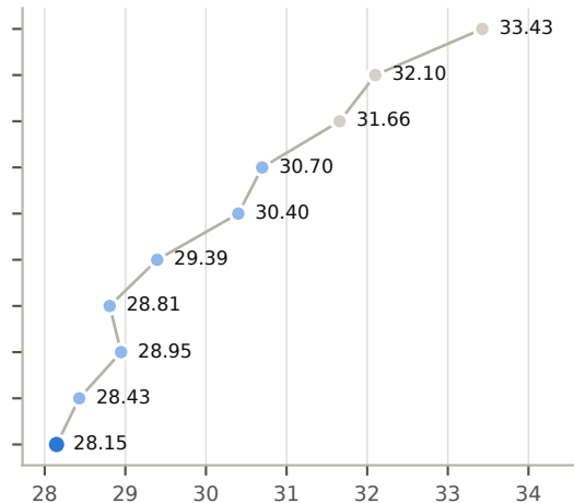
CRPS~ (AUD/MWh)
