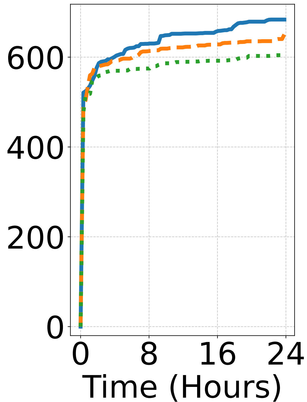
HDFS
