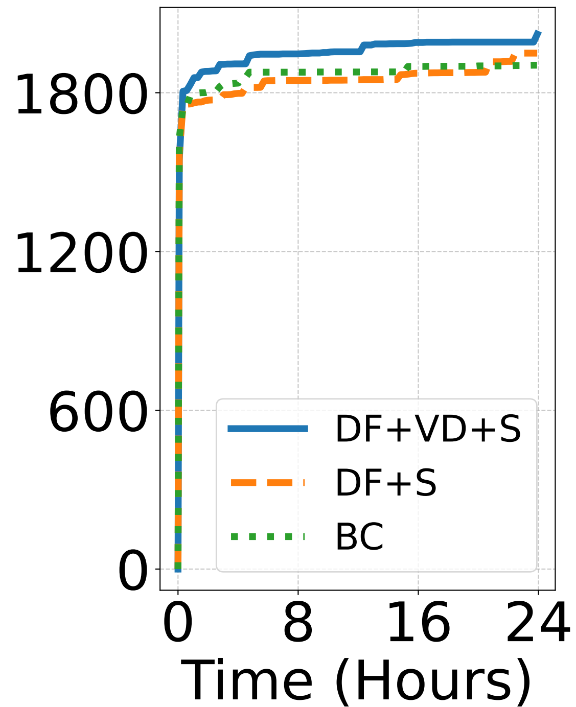
HBase
