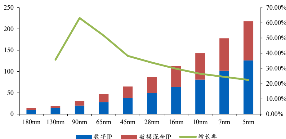
图表 19 不同工艺节点下的芯片所集成的硬件 IP 平均数量
