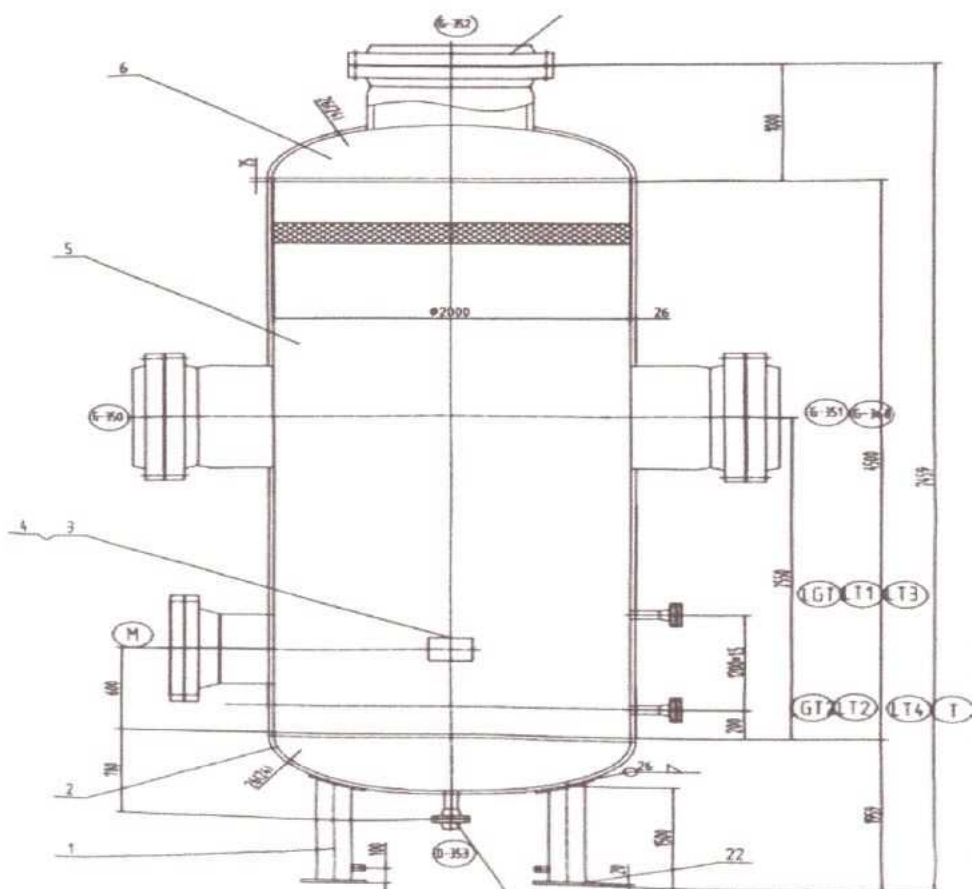
图 3 1#分离器结构图
