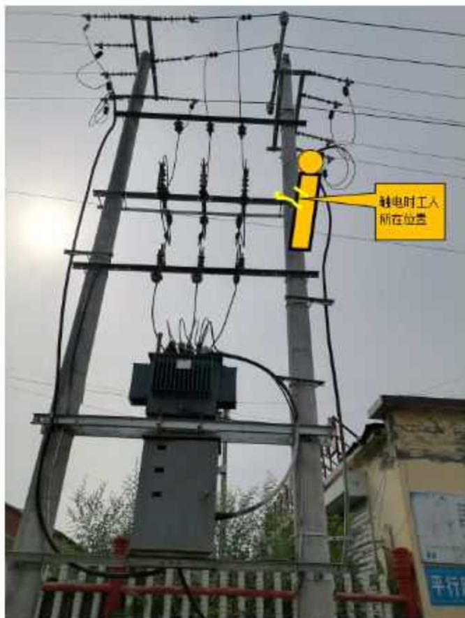
图 2 施工人员触电位置示意图（跌落开关上口带电 10KV）
