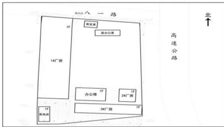
厂区图
